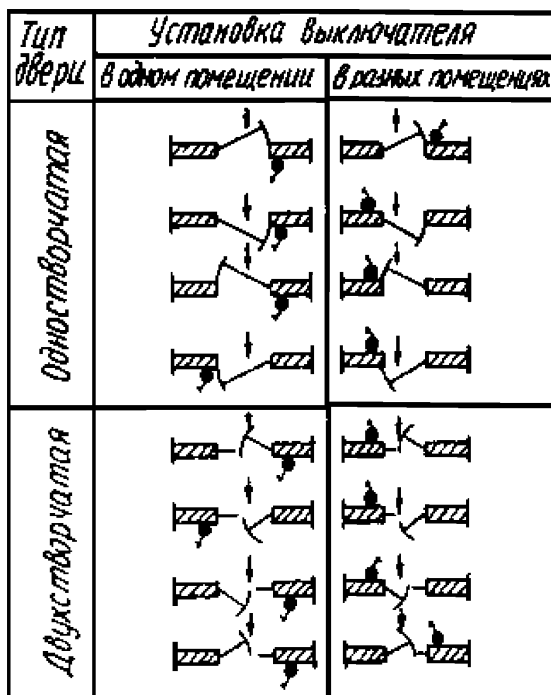
Рис.21. Места установки выключателей в помещениях
