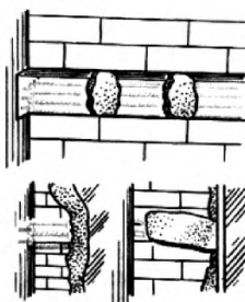
Рис.3. Скрытые электропроводки под негорючими основаниями
