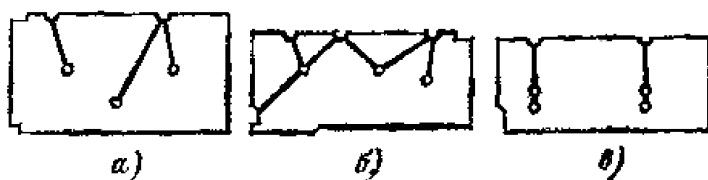
Рис.13. Примеры выполнения каналов в железобетонных панелях перекрытий (а, б) и стеновой панели (в)
