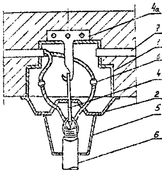
Рис.43. Замоноличенная потолочная коробка
