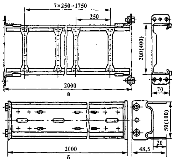
Рис.1. Металлические прямые лотки:
