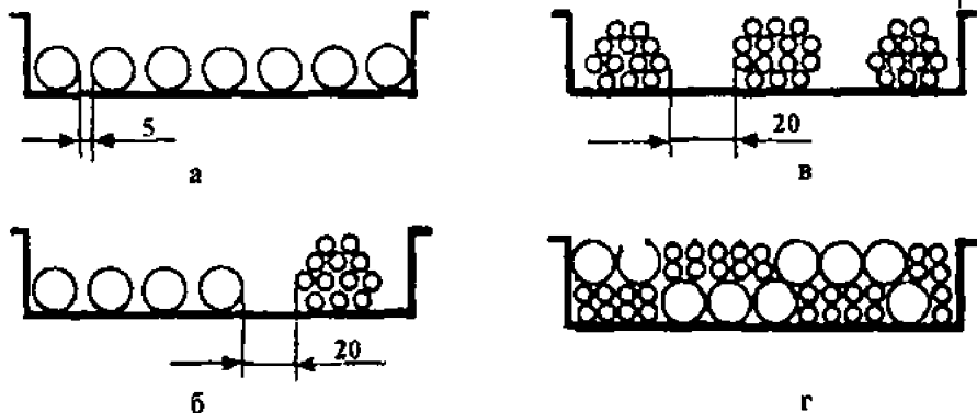
Рис.2. Способы прокладки проводов и кабелей на лотках:
