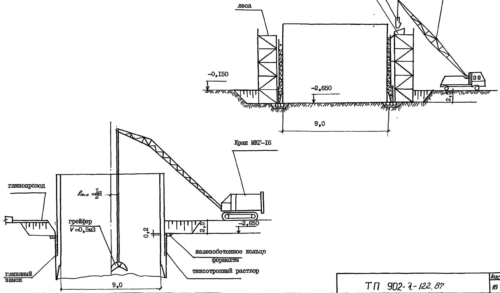
Схема погружения ошускного колодца в связных грунтах
