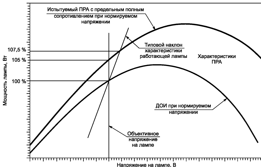
Рисунок D.1 — Характеристики соответствия настройки ПРА для натриевой лампы высокого давления, работающей с ДООИ и испытуемым ПРА при номинальном напряжении питания
