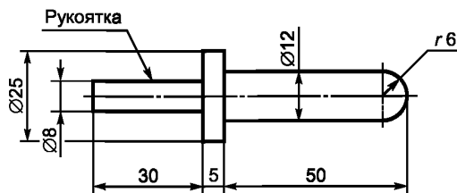
Рисунок 101 — Испытательный щуп «а»
