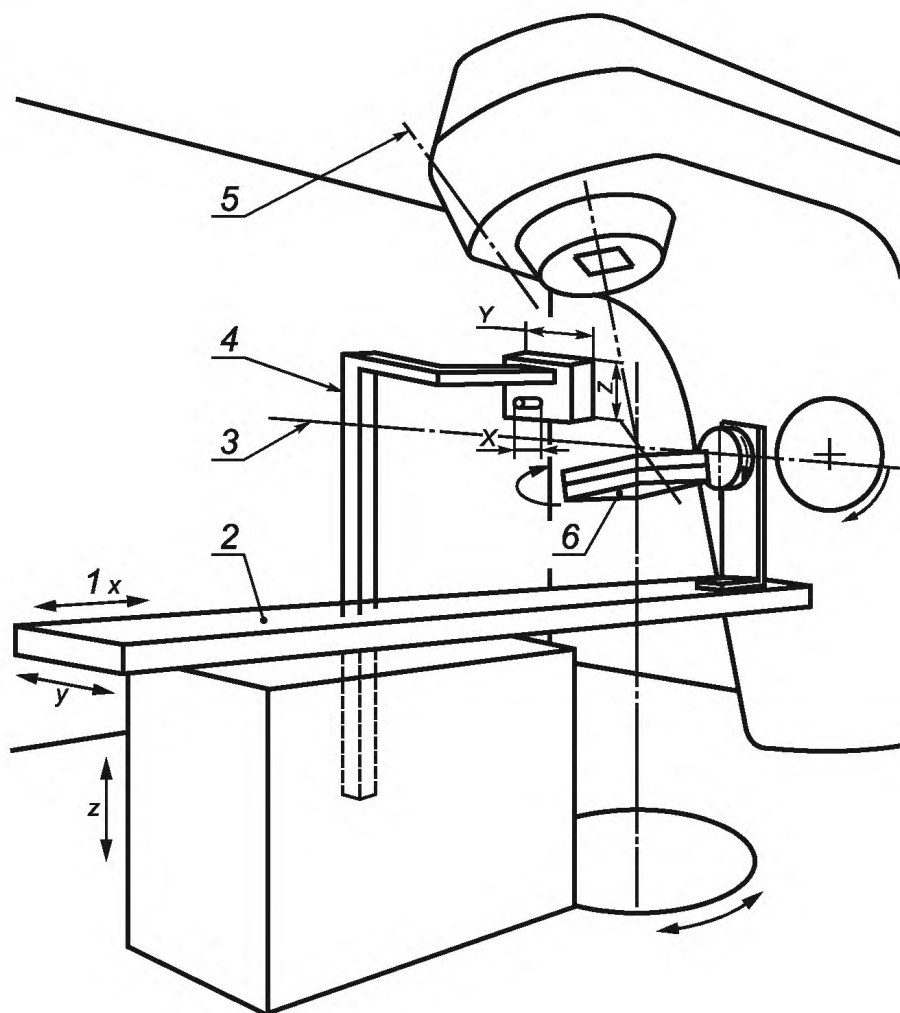
1 — x , y , z — микрометрическая настройка опорного указателя; 2 — дека СТОЛА для ПАЦИЕНТА; 3 — настенный источник света; 4 — держатель центратора, укрепленный на полу, позволяющий поворачивать ШТАТИВ на 360^\circ и СТОЛ для ПАЦИЕНТА на меньшие углы; 5 — потолочный источник света; 6 — блок из моделирующего материала и пленка
