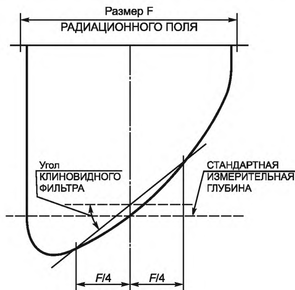
Рисунок 7 — Пояснение к определению УГЛА КЛИНОВИДНОГО ФИЛЬТРА
