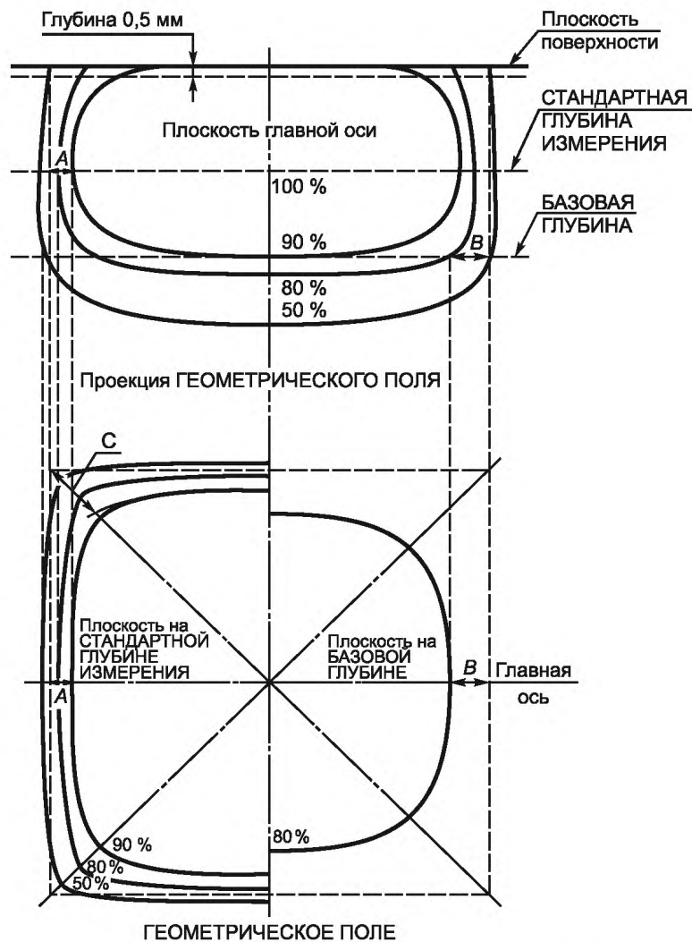
Рисунок 6 — Примеры диаграммы равномерности ЭЛЕКТРОННОГО ПОЛЯ Значения С определяют вдоль диагональных осей; для неквадратных РАДИАЦИОННЫХ ПОЛЕЙ — не по биссектрисе
