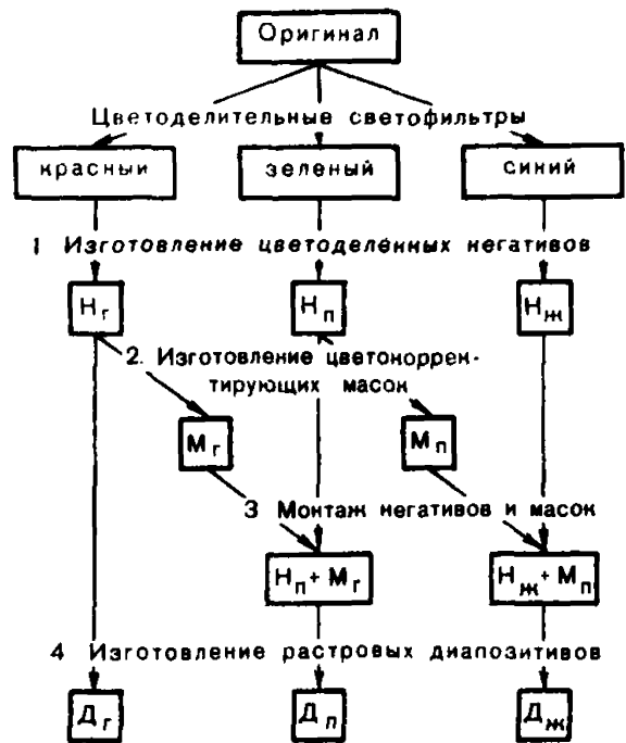
Рис. 10. Схема перекрестного (одно-ступенчатого) маскирования
