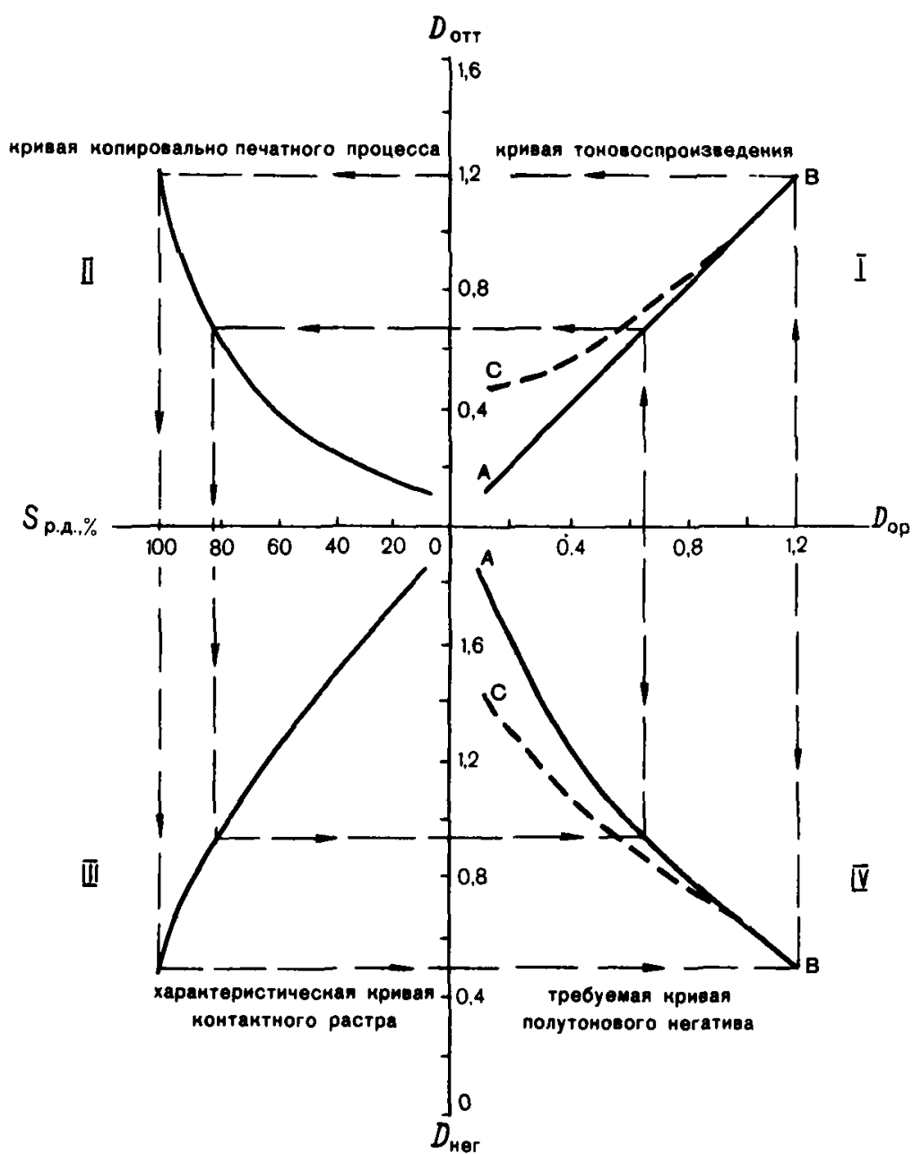
Рис. 6. Схема графического построения для определения требуемой градационной кривой полутонового негатива
