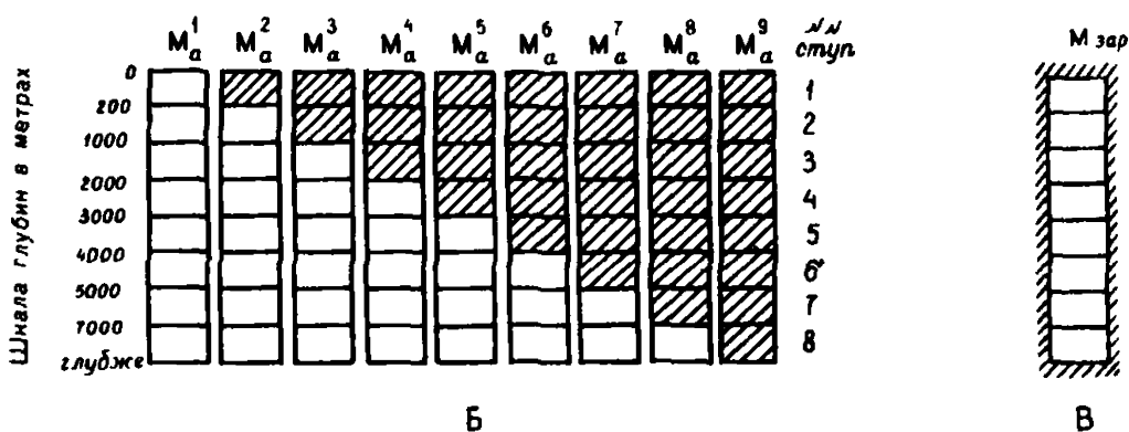
Рис. 19. Схема изготовления перекрывающихся масок ступеней послойной окраски для воспроизведения физико-географических карт: А — маски ступеней гипсометрической окраски; Б — маски ступеней окраски акваторий; В — маска зарамочная
