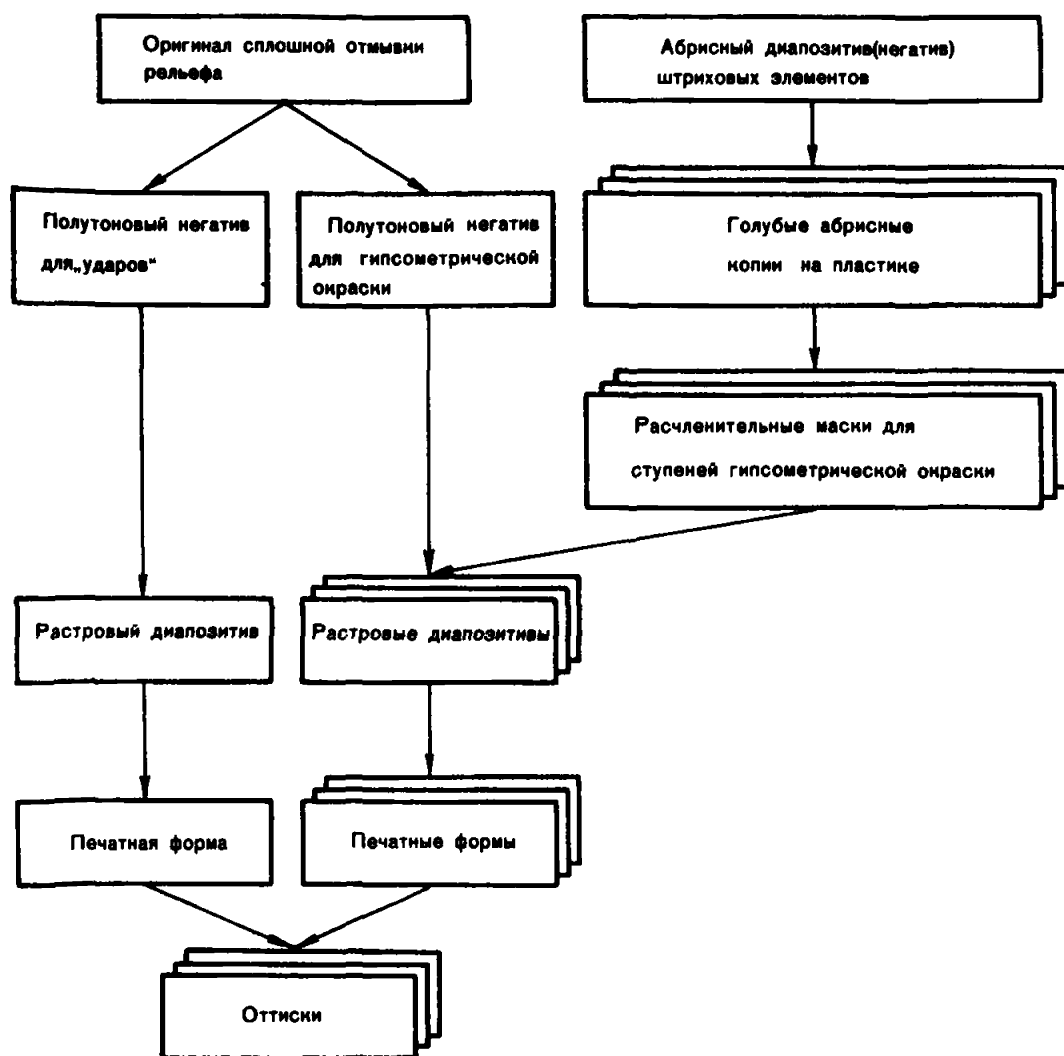
Рис. 18. Схема технологических процессов воспроизведения изображения рельефа на физико-географических картах с применением оригинала сплошной отливки рельефа и расчленительных масок
