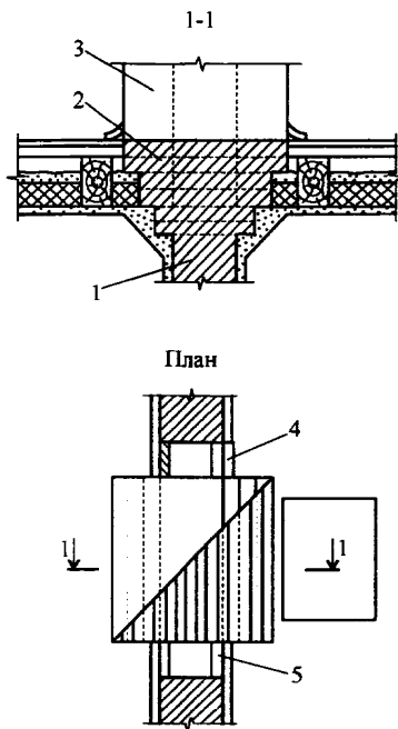
Рис. 3.6. Основание печи на уширении стены: 1 - стена; 2 - основание печи; 3 - печь; 4 - вентиляционная решетка; 5 - разделка из кирпича.
