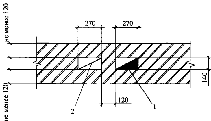
Рис. 6.1. Размещение каналов во внутренней стене: 1 - дымовой канал; 2 - вентиляционный канал.
