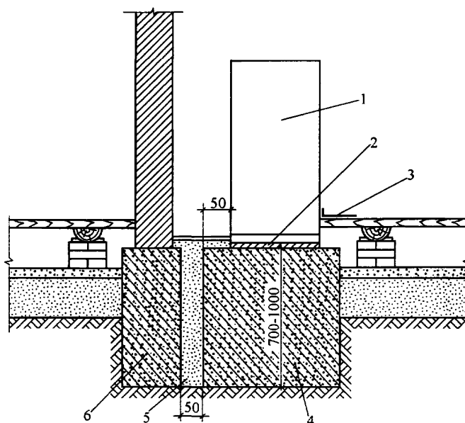
Рис. 3.4. Размещение печи на отдельном фундаменте: 1 - печь; 2 - гидроизоляция; 3 - предтопочный лист; 4 - фундамент печи; 5 - засыпка; 6 - фундамент стены.
