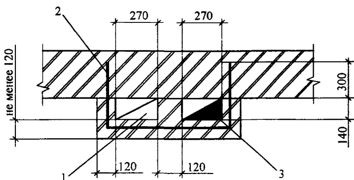
Рис. 6.2. Пристроенные каналы к внутренней кирпичной стене: 1 - вентиляционный канал; 2 - анкерный стержень на 1 м высоты через 6 рядов кладки; 3 - дымовой канал.
