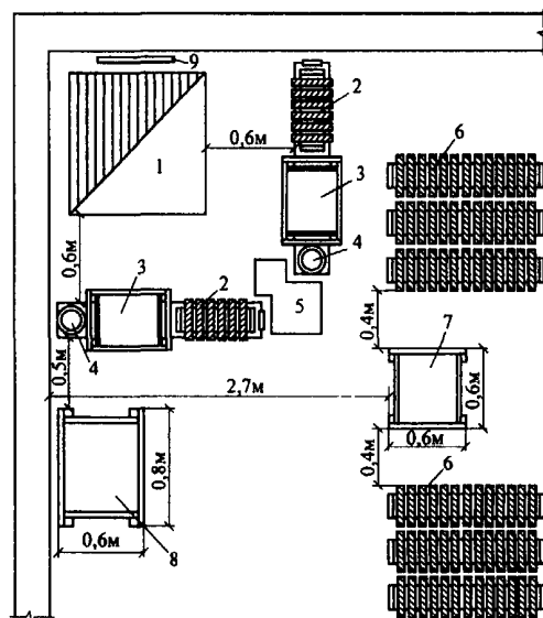
Рис. 2.1. Схема организации рабочего места при кладке печи у стены и в углу помещения: 1 - печь; 2 - рама с кирпичом; 3 - ящик с глиной; 4 - ведро; 5 - кирпич ломаный, кирпич огнеупорный, изразцы; 6 - запас кирпича; 7 - емкость с водой для замачивания кирпича; 8 - ящик с раствором; 9 - рама с чертежом.
