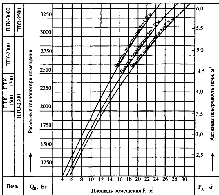
Рис. 3.2. Номограмма для определения теплотер угловых комнат
