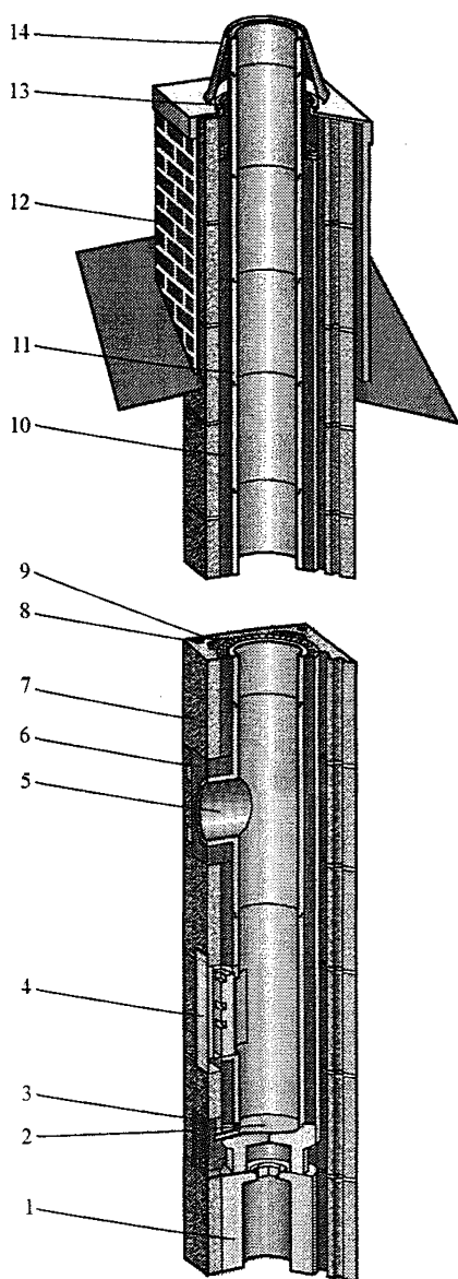
Рис. 6.8. Конструкция керамической дымовой трубы:
