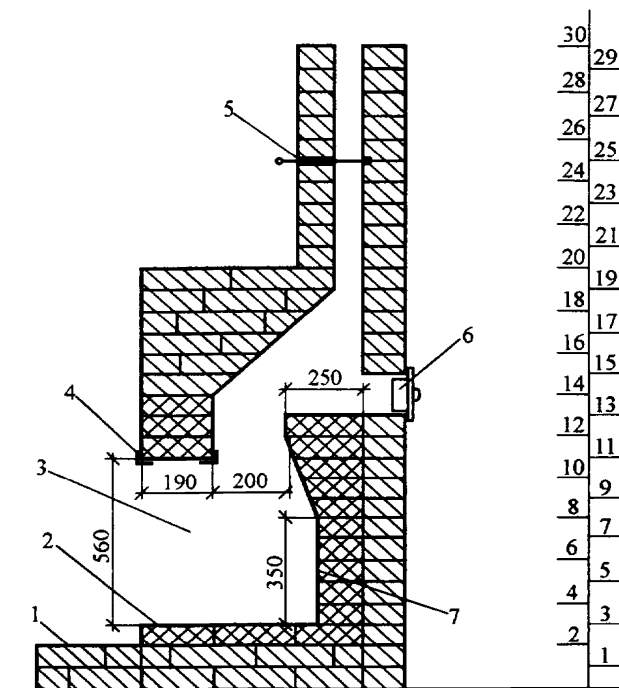
Рис. 5.1. Устройство камина из кирпича: 1 - площадка; 2 - под топки; 3 - топливник; 4 - уголок; 5 - задвижка; 6 - устройство для чистки; 7 - задняя стенка топливника.
