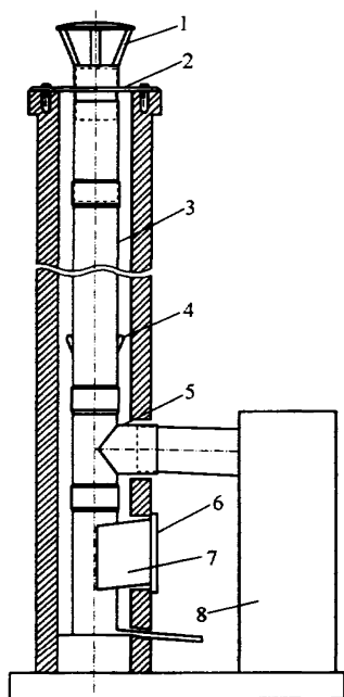
Рис. 6.6. Прокладка трубы в кирпичном канале: 1 - зонт; 2 - кровельная плита; 3 - металлическая труба; 4 - монтажные зацепы; 5 - тройник; 6 - дверка; 7 - очистной люк с отводом конденсата; 8 - теплогенератор.
