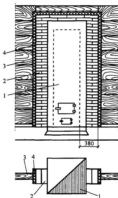
Рис. 3.9. Устройство вертикальной разделки: 1 - печь; 2 - вертикальная разделка; 3 - сгораемая конструкция; 4 - теплоизоляция.
