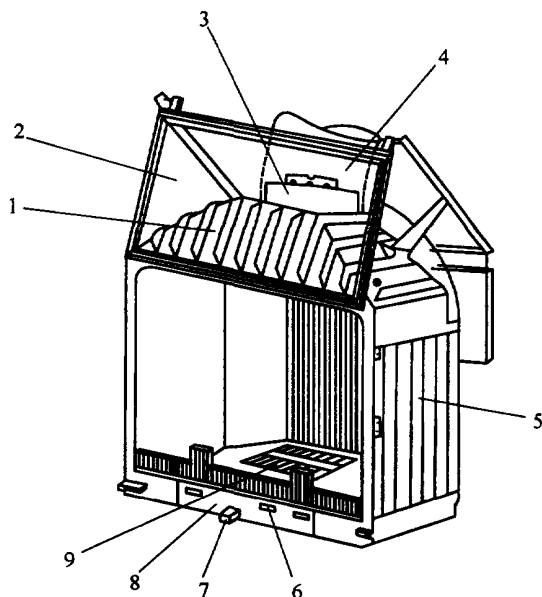
Рис. 5.3. Общий вид топки камина:
