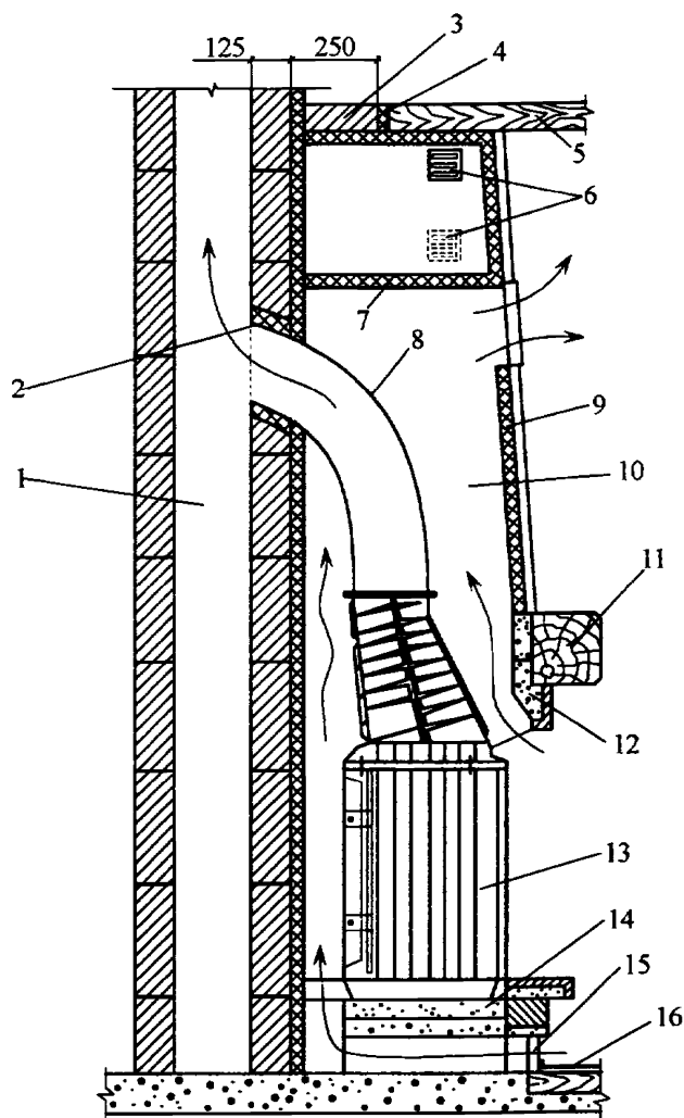
Рис. 5.4. Устройство камина закрытого типа: 1 - дымовой канал; 2 - уплотнительное устройство; 3 - противопожарная раздела; 4 - теплоизоляция для защиты конструкции от возгорания; 5 - деревянная конструкция; 6 - решетка; 7 - защитный экран; 8 - дымоотвод; 9 - теплоизоляция; 10 - защитный кожух; 11 - полка; 12 - пояс жесткости; 13 - камин; 14 - основание; 15 - отверстие для поступления воздуха; 16 - предпочный лист.
