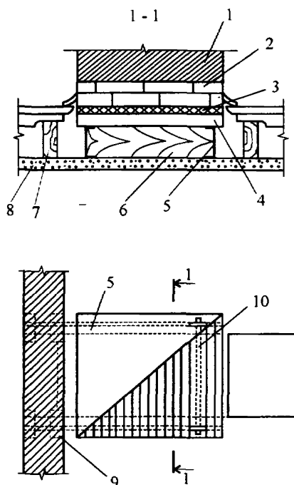
Рис. 3.5. Основание печи на консолях:
