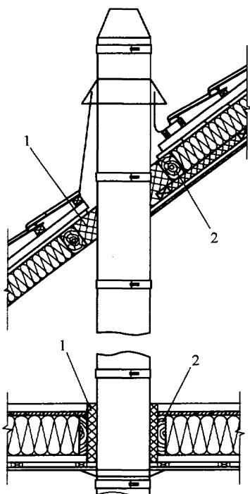
Рис. 6.14. Схема противопожарной разделки: 1 - теплоизоляция; 2 - деревянные конструкции.
