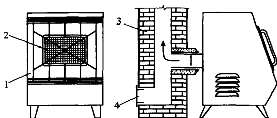
Рис. 5.2. Газовый камин:
