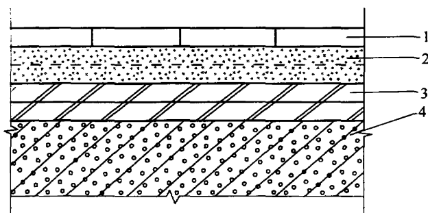
Рис. 5.5. Детали пола:
