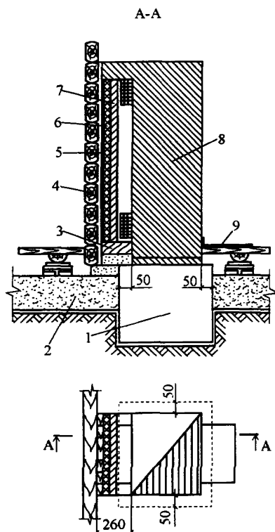
Рис. 3.8. Устройство закрытой отступки: 1 - фундамент печи; 2 - уплотнительный слой; 3 - негоряемый пол; 4 - деревянная стена; 5 - щит из досок; 6 - теплоизоляция (асбест или войлок); 7 - кирпич "на ребро"; 8 - печь; 9 - предтопочный лист.
