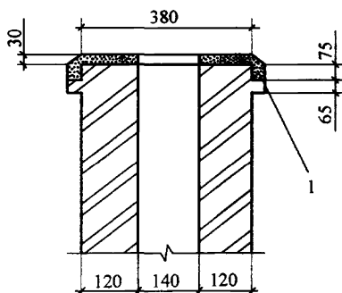
Рис. 6.5. Устройство оголовка: 1 - цементно-песчаный раствор состава 1:2.
