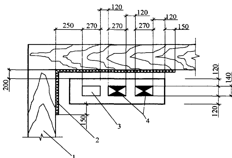
Рис. 6.11. Устройство отступки:
