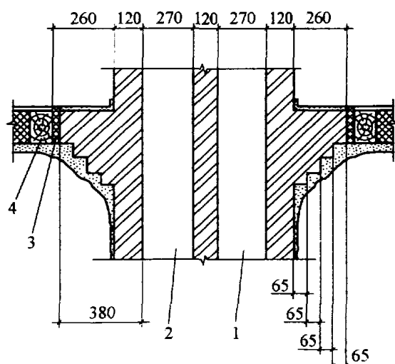
Рис. 6.12. Горизонтальная разделка:
