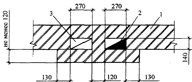
Рис. 6.3. Размещение каналов в наружной кирпичной стене: 1 - наружная поверхность; 2 - дымовой канал; 3 - вентиляционный канал.
