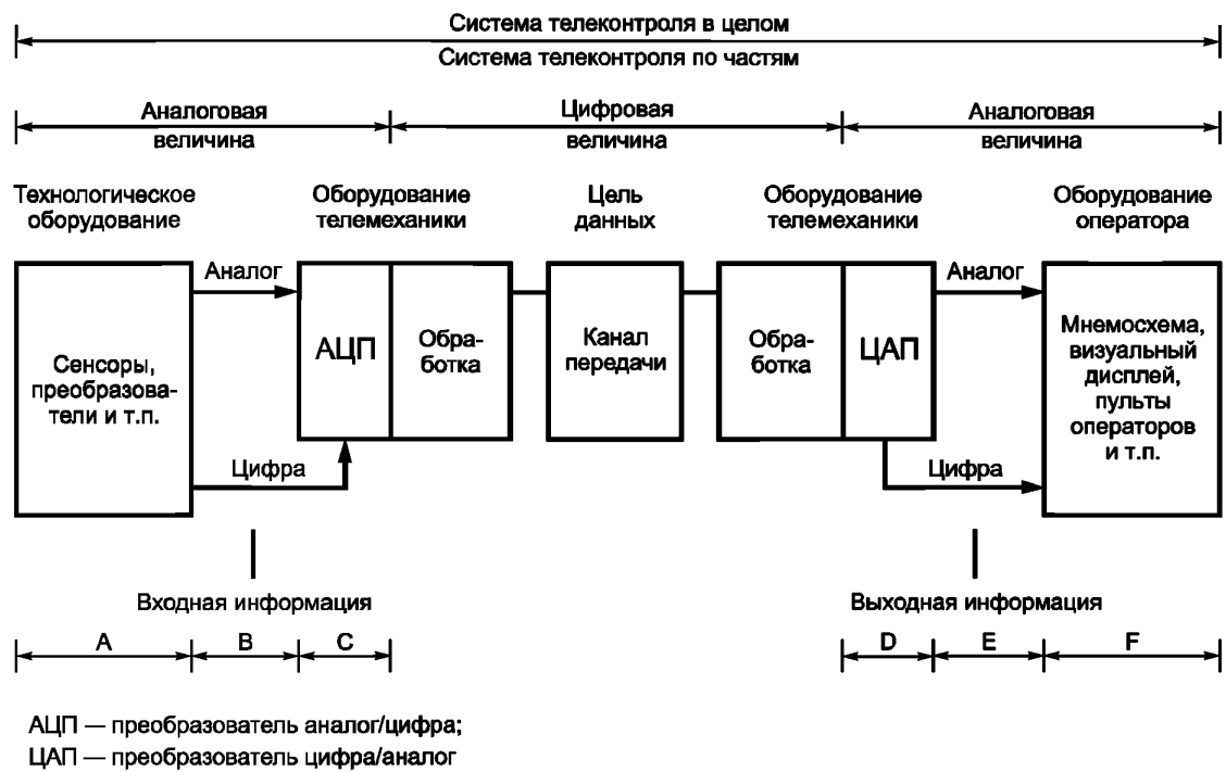
Рисунок 1 — Обработка аналоговой информации
