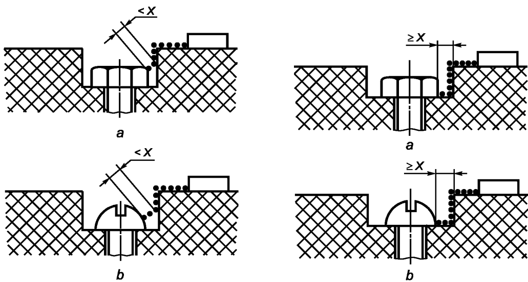
Зазор между головкой винта и стенкой углубления имеет недостаточные размеры для того, чтобы его учитывать при измерении путей утечки. Зазор между головкой винта и стенкой углубления имеет достаточные размеры, для того, чтобы его учитывать при измерении путей утечки.
