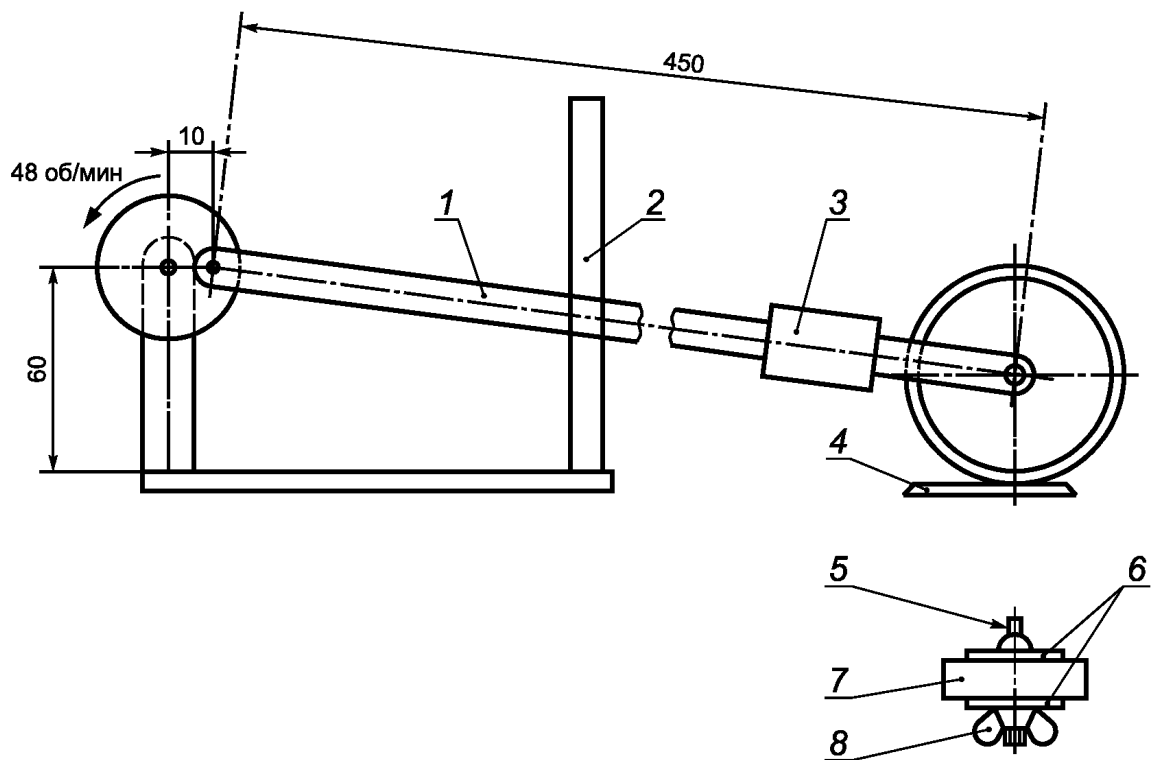
1 — полоса из мягкой стали 25 × 5; 2 — направляющая для полосы; 3 — подвижный груз; 4 — образец; 5 — крюк для пружинных весов; 6 — латунная шайба 60 × 2,5; 7 — твердый белый полировочный войлок 65 × 7,5; 8 — гайка «барашек»
