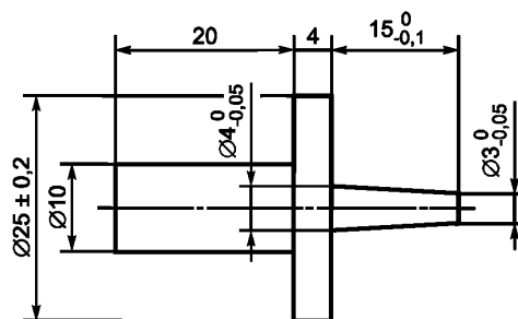
Рисунок 1 — Испытательный стержень
