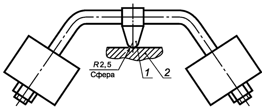
1 — сферическая часть; 2 — образец
