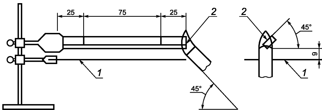
1 — тканая проволоочная сетка; 2 — образец
