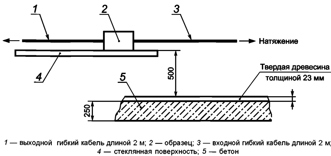
Рисунок 4 — Испытание на удар отдельно стоящих управляющих устройств
