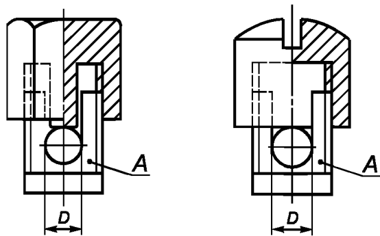
A — закрепленная часть; D — пространство для провода
