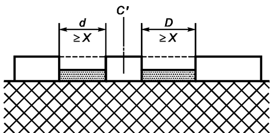
C' — подвижная часть. Воздушный зазор составляет расстояние d + D . Расстояние пути утечки также составляет d + D .
