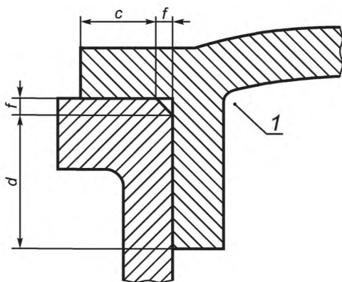
Рисунок 2а — Цилиндрическая часть
