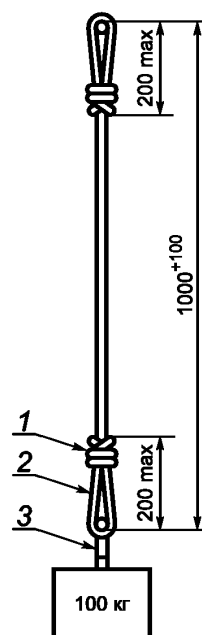
1 — узел; 2 — оконечная петля; 3 — точка присоединения
