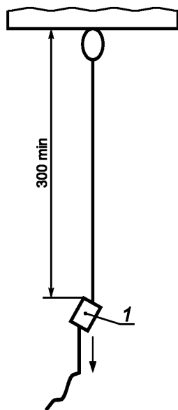
1 — устройство позиционирования на канатах
