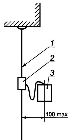
1 — анкерный канат; 2 — устройство позиционирования на канатах; 3 — груз массой 5 кг
