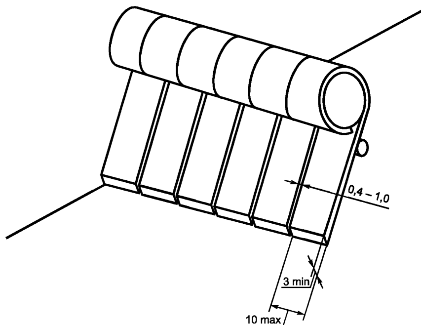
Рисунок 3 — Размеры захватывающего элемента
