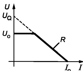
Рисунок С.1b — Трапециевидная характеристика
