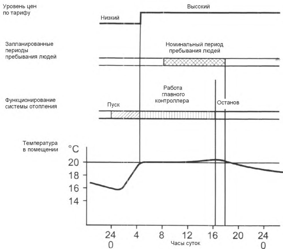
Рисунок 3 — Оптимизатор с компенсацией тарифа для минимизации затрат (сдвигает начало пускового периода на конец периода с пониженным тарифом)
