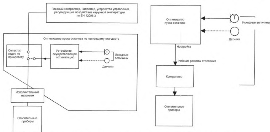
Рисунок 4 — Примеры применения оптимизатора пуска-останова
