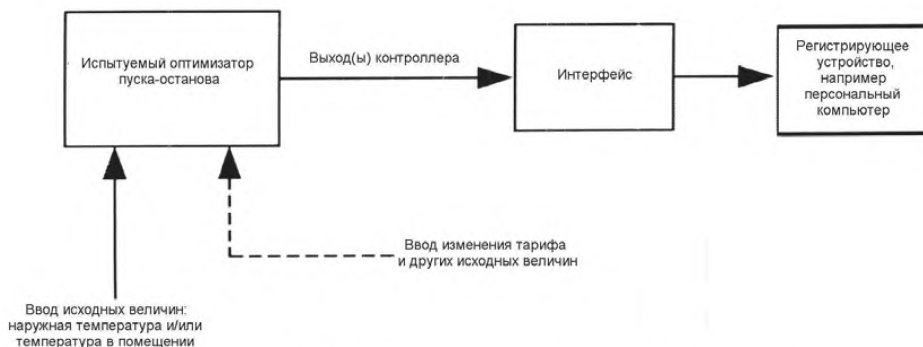
Рисунок 15 — Пример блок-схемы испытательной установки
