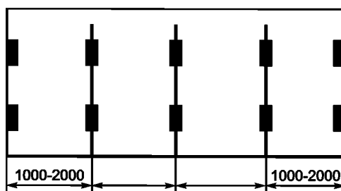
Рисунок В.3 — Размещение пяти пар опорных площадок
