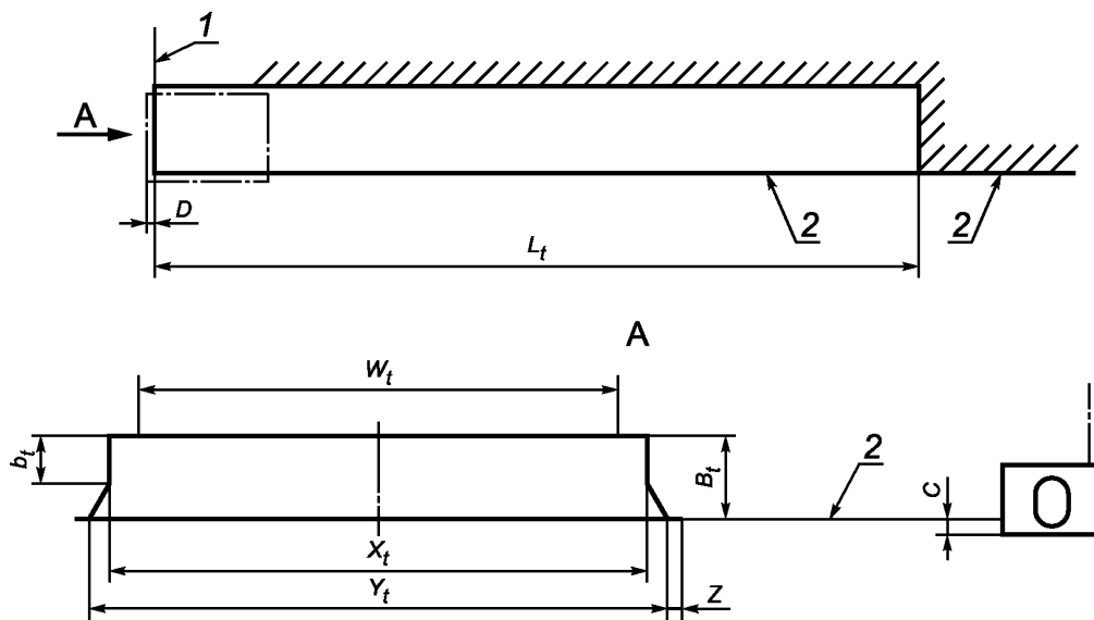
Рисунок Е.1 — Размеры тоннеля контейнера, в который может войти балка типа «шея гуся» полуприцепа
