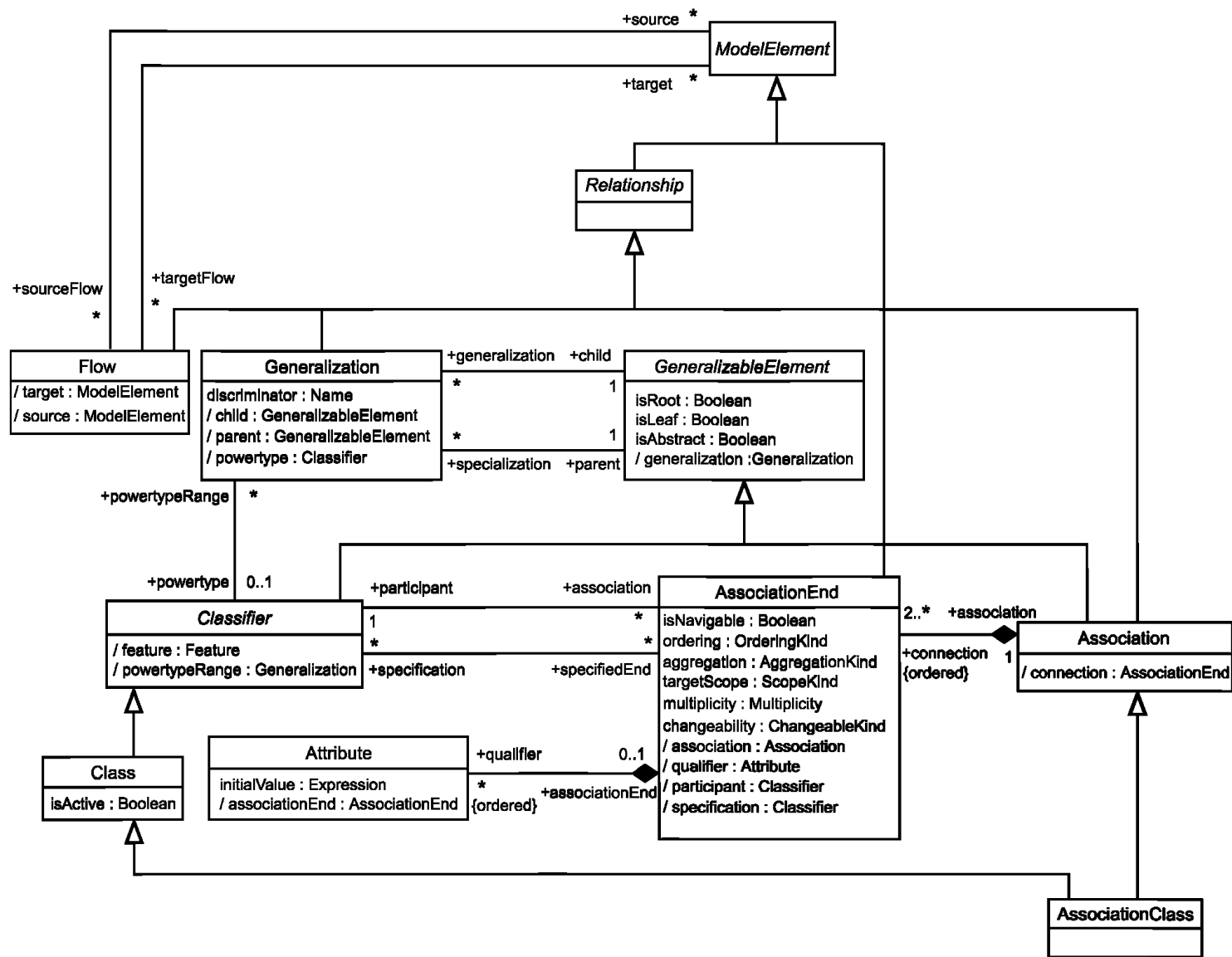
Рисунок D.2 — Главный пакет — Взаимосвязи (рисунок 5-3 из [4])
