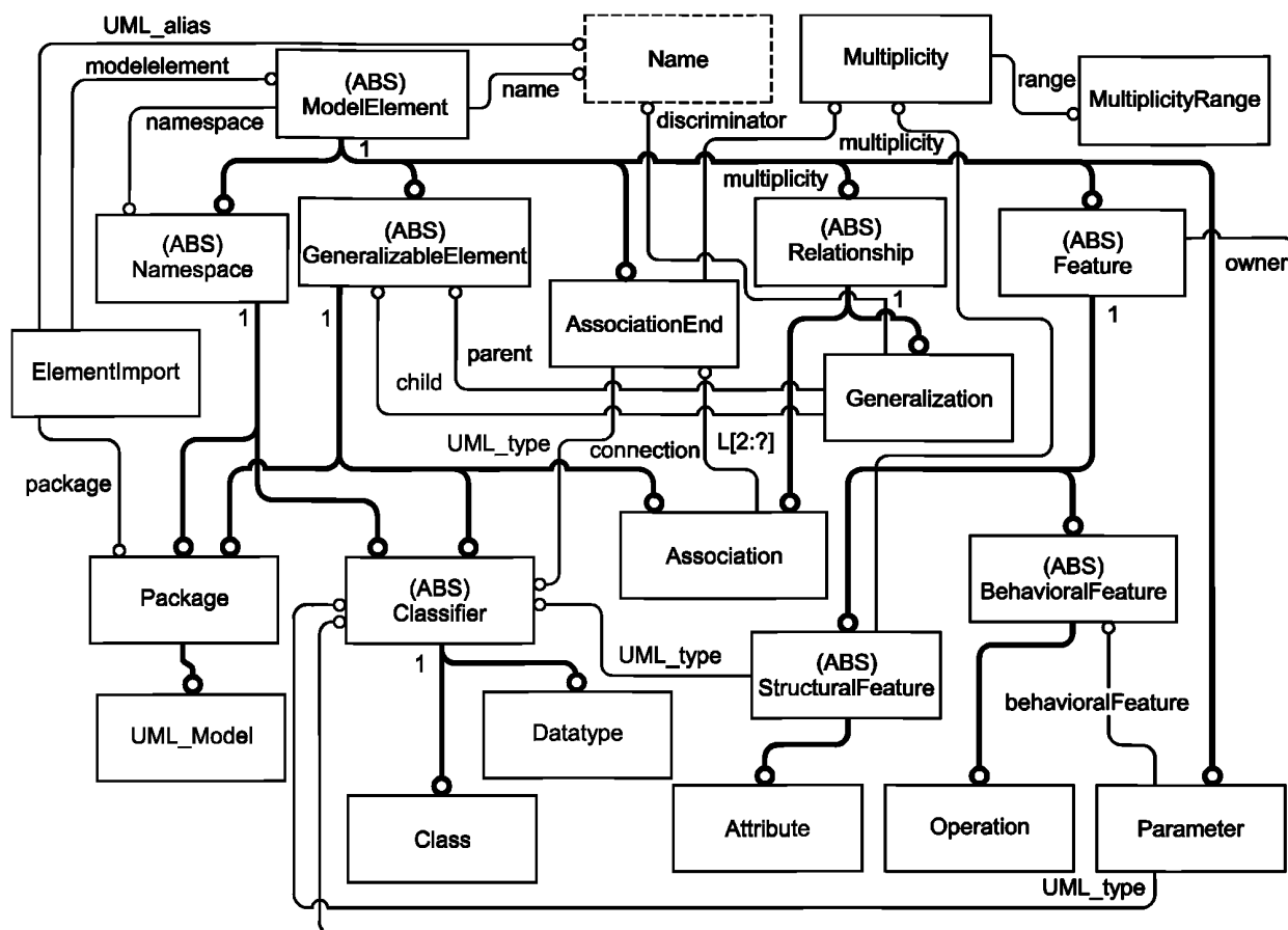
Рисунок 4 — EXPRESS-G диаграмма частей метамодели обмена UML
