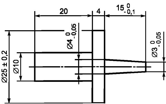
Рисунок 2 — Испытательный щуп
