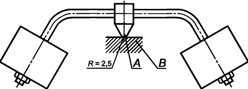
Рисунок 5 — Испытательное устройство для вдавливания шарика
