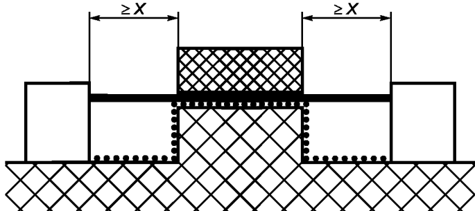
Рисунок E.5 — Неплошной стык с узкими канавками
