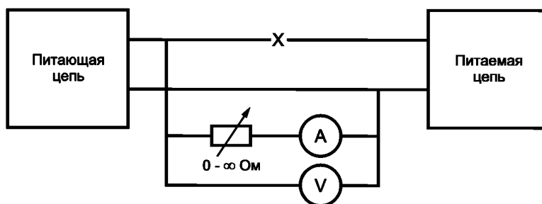
Рисунок 1 — Схема испытательной цепи для условий неисправности
