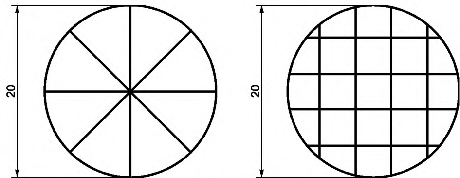
Рисунок 12 — Образец царапин для испытаний на взрывоопасность
