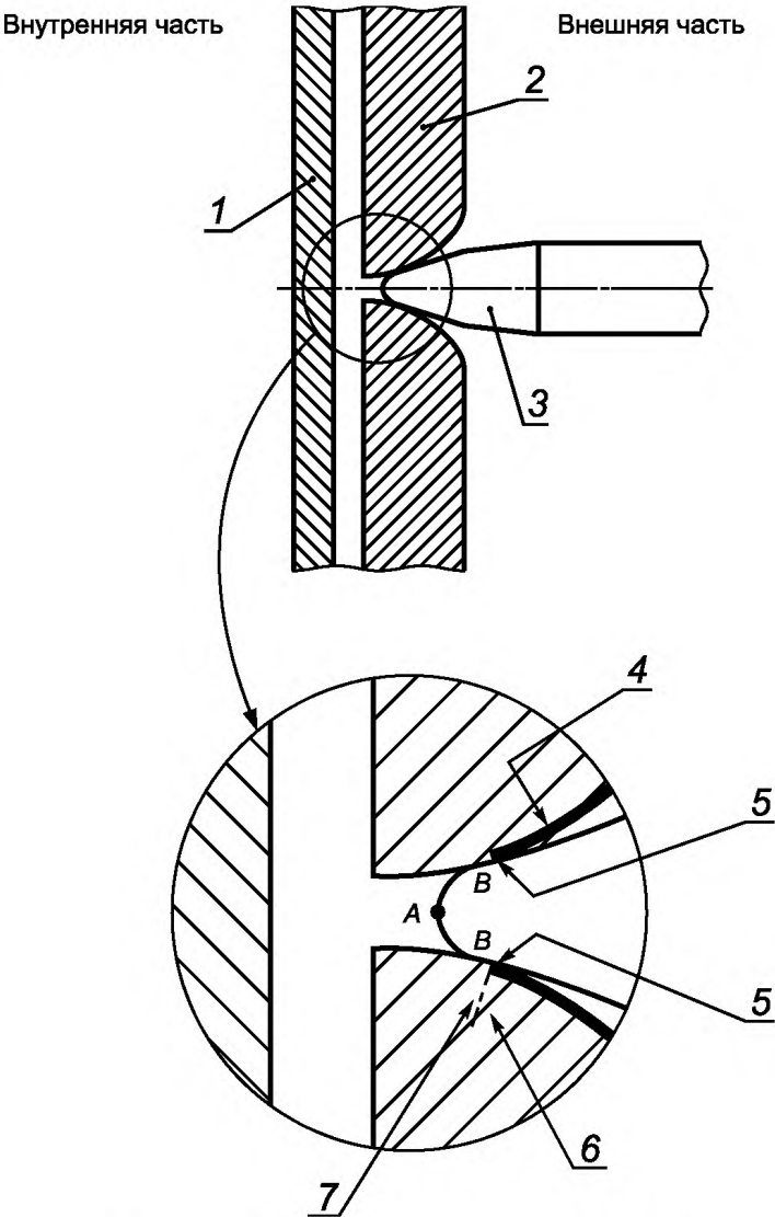
1 — часть под опасным напряжением; 2 — корпус из изоляционного материала; 3 — испытательный палец; 4 — поверхность, считающаяся покрытой металлической фольгой; 5 — точка контакта; 6 — доступная для испытательного пальца поверхность; 7 — недоступная для испытательного пальца поверхность
