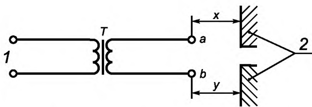
1 — сеть питания; 2 — электрически разделенные доступные проводящие части
