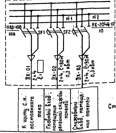
Схема щитка аварийного освещения ЩС ЯОУ-8504
