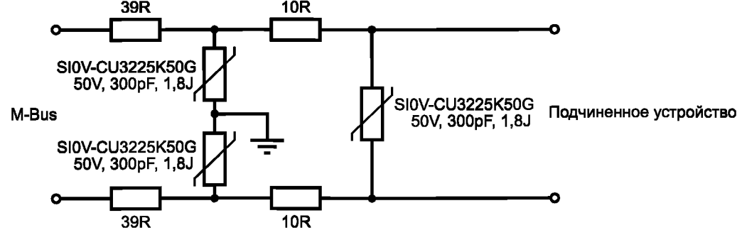
Рисунок Е.6 — С заземлением (100 × 2 кВ × 50 мкс)
