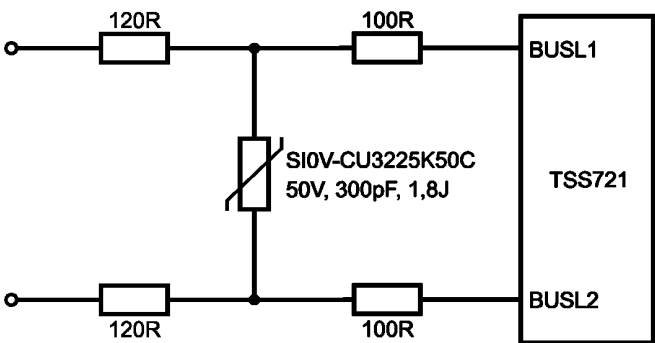
Рисунок Е.1 — Без заземления (100 × 6 кВ × 50 мкс)
