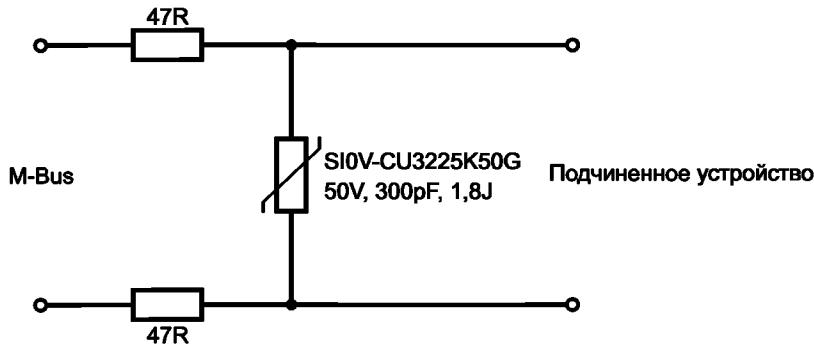
Рисунок Е.5 — Без заземления (100 × 2 кВ × 50 мкс)
