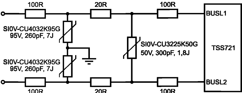
Рисунок Е.2 — С заземлением (100 × 6 кВ × 50 мкс)
