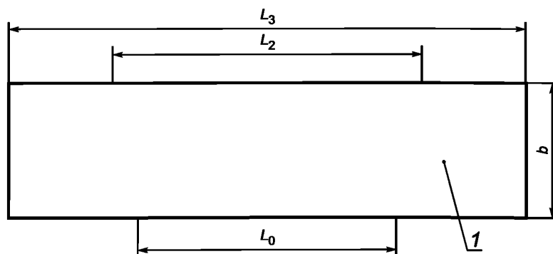
Рисунок 1 — Образец-полоска (метод А)
