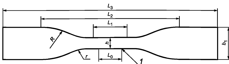
Рисунок 2 — Образец-лопатка (метод В)
