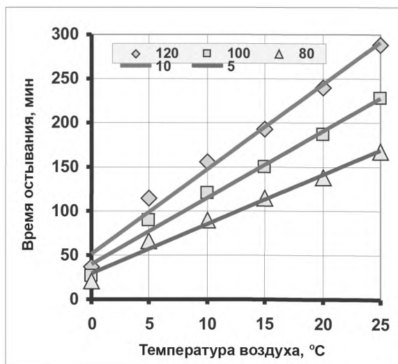
Рисунок В.2 – Время остывания холодной асфальтобетонной смеси до температуры 25 °С (в зависимости от температуры выпуска смеси из асфальтосмесителя)
