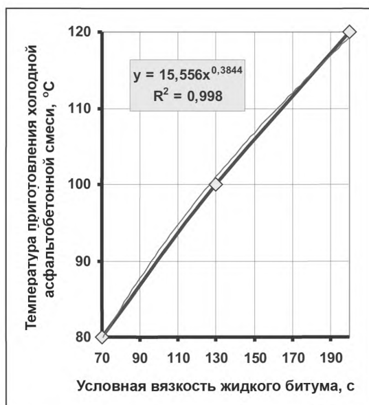
Рисунок В.1 – Температура приготовления холодной асфальтобетонной смеси
