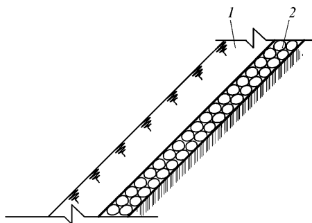
Рисунок 2 – Пример заполнения коробчатых габрионных конструкций растительным грунтом
