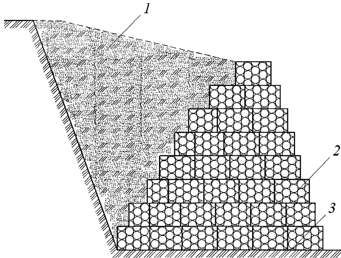
1 – обратная засыпка; 2 – коробчатый габион; 3 – основание сооружения
