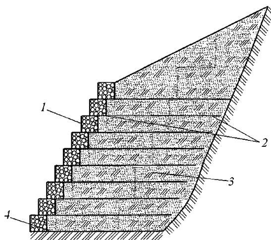
1 – ступенчатая лицевая грань сооружения; 2 – коробчатый габион с армирующей панелью; 3 – обратная засыпка; 4 – основание сооружения
