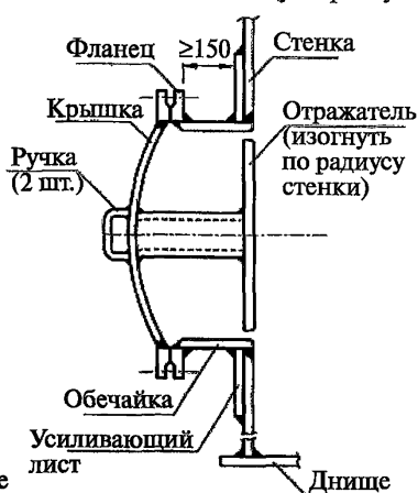
Рис. 19. Люки-лазы в стенке резервуара. Разрезы
