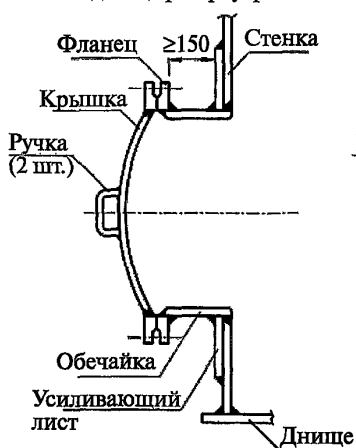
Рис. 19. Люки-лазы в стенке резервуара. Разрезы
