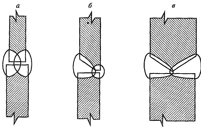
Рис. 3. Горизонтальные стыковые соединения стенки:
