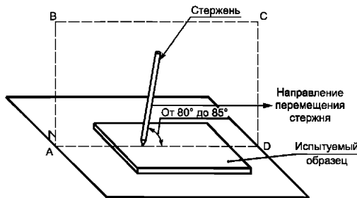
Стержень находится в плоскости ABCD, перпендикулярной плоскости образца Рисунок 103 — Испытание на прочность покрытия оболочки блока питания царапанием
