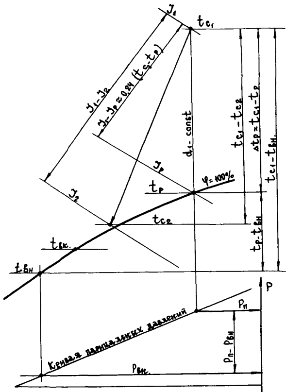
Рис.3 Графическая интерпретация расчетных величин \Delta J ; \Delta T_c ; M_1 ; R и \alpha в U-d - диаграмме.
