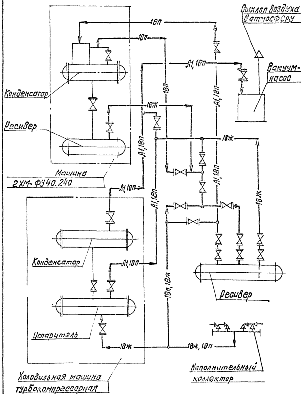
Рис. 9 Схема подключения 2ХМ-ФУ40.240 к холодильной станции с турбомашинami по схеме ресиверной станции Казанского компрессорного завода
