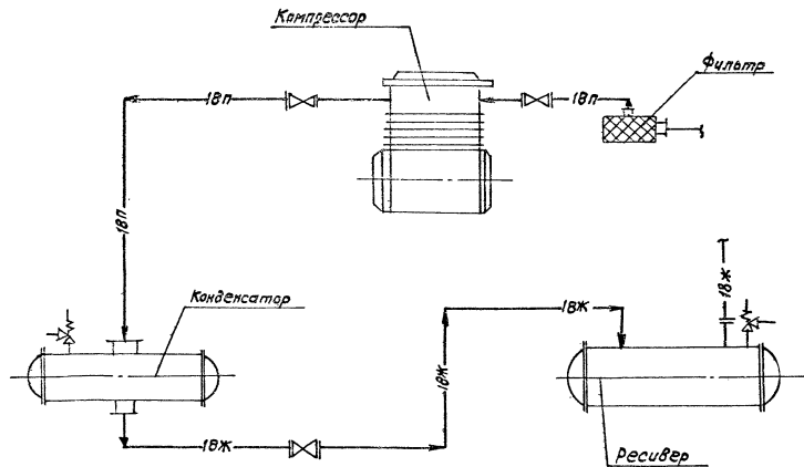
Рис.5 Принципиальная схема машины 2XM-ФУ40.240
