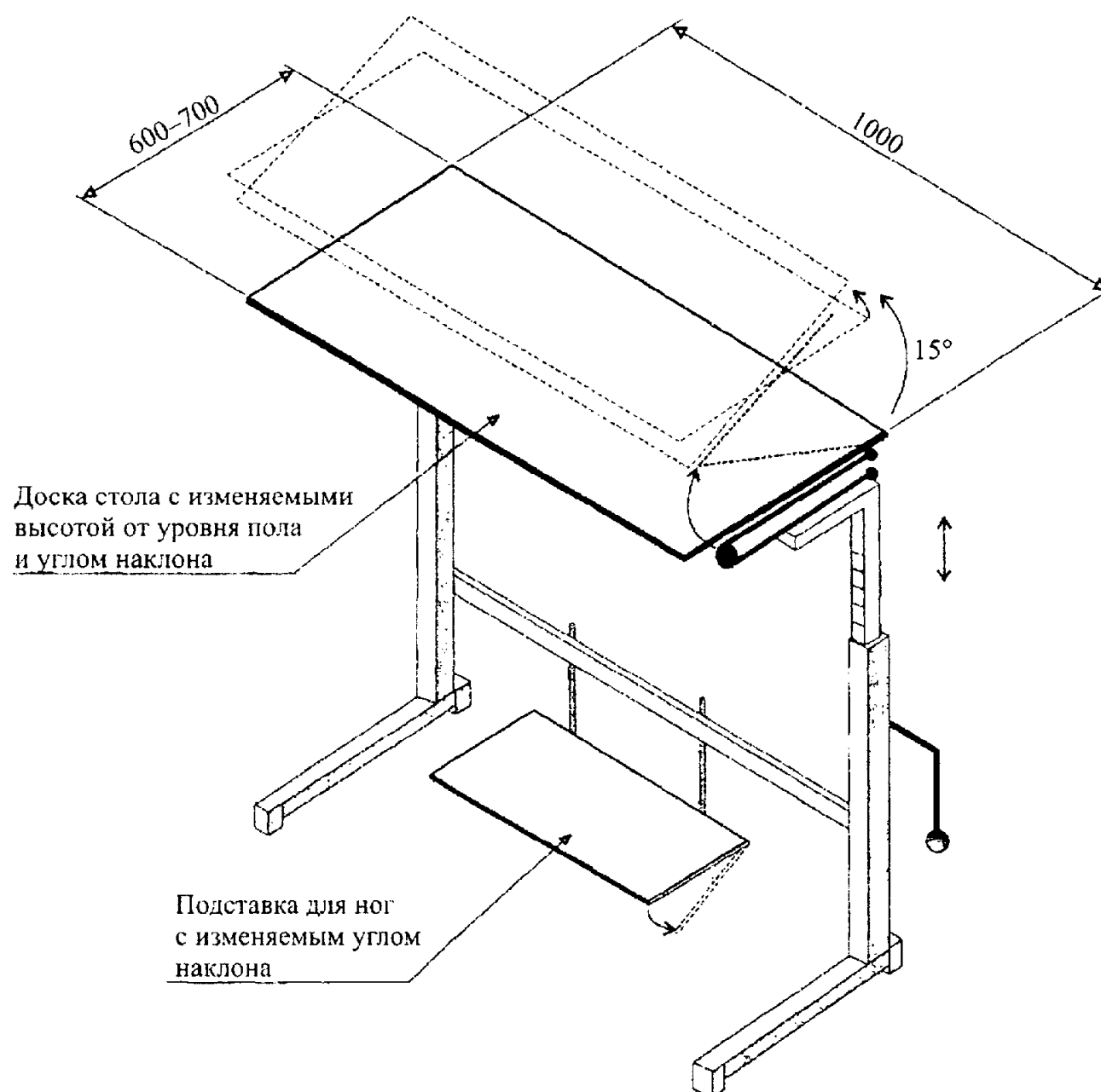
Рисунок В.12 – Трансформируемый рабочий стол для инвалида
