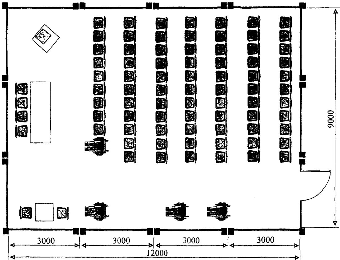
Места инвалидных колясок в помещении для собраний
