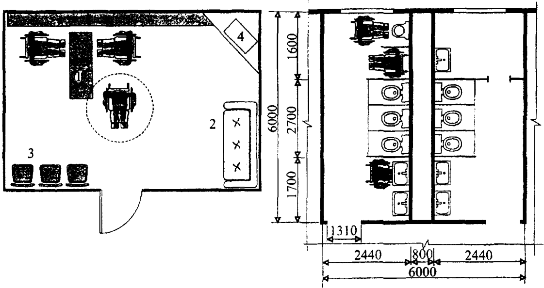
Встроенное помещение инвентарного типа для пассивного отдыха; пример оборудования комнаты отдыха для инвалидов: 1 – стол для настольных игр; 2 – диван; 3 – кресла; 4 – телевизор
