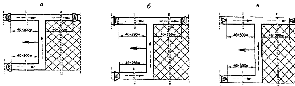
Рис. 5. Схемы установки заслонов от сопряжения с очистной выработкой в конвейерной выработке и в вентиляционной выработке, по которой отводится вентиляционная струя при прямоточных с подсвежением схемах проветривания
