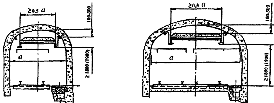
Рис. 4. Схема установки сланцевых заслонов в выработках, закрепленных бетонной крепью
