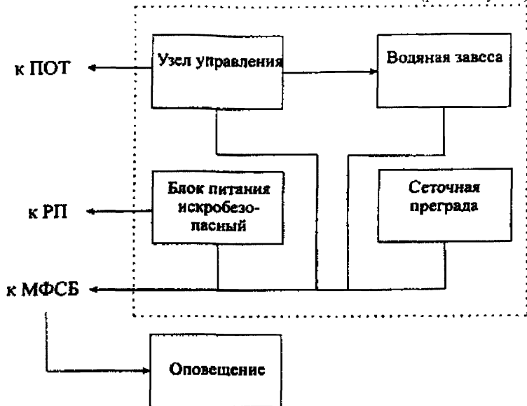
Рис. 1. Блок-схема подключения АВЗ:
