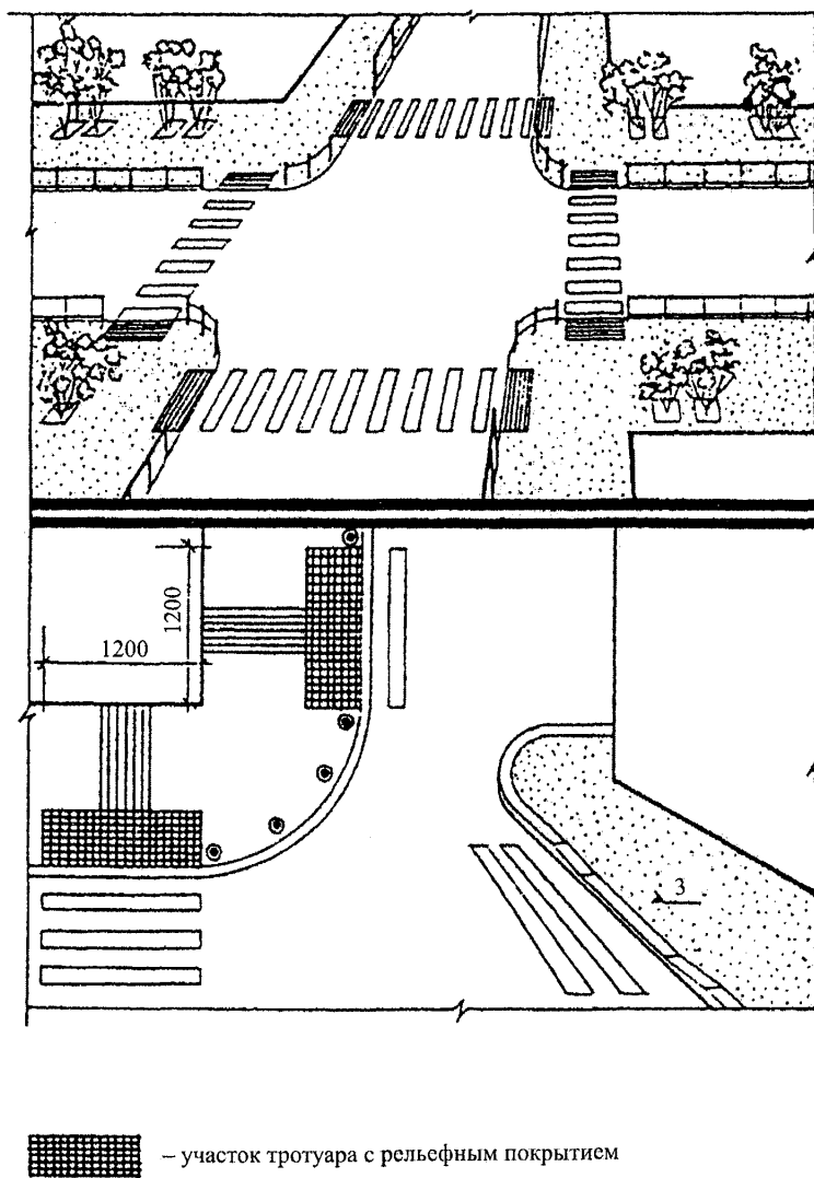
Рисунок В.8 – Устройство переходов через внутризаводские проезды
