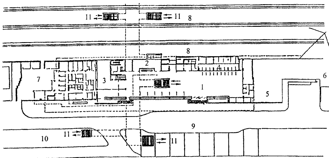
План первого этажа
