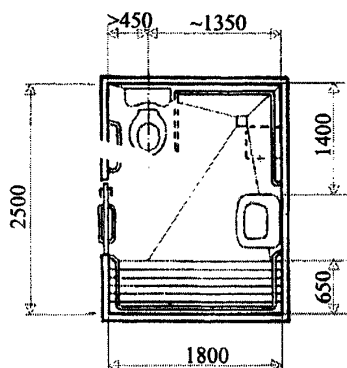
Непроходная кабина
