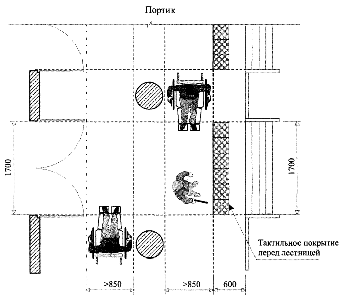
Рисунок В.16 – Площадки перед тамбуром и портиком
