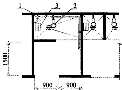
Душевая кабина для инвалида на кресле-коляске
