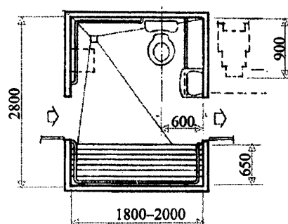
Вариант конструкции сиденья в душевой
