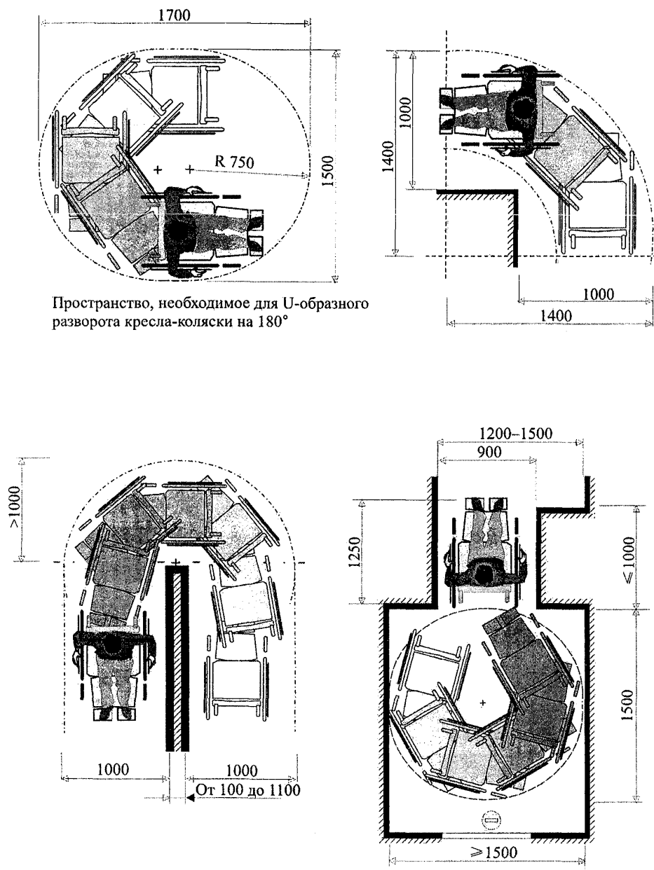
Рисунок В.9 – Габариты поворотов и разворотов кресла-коляски
