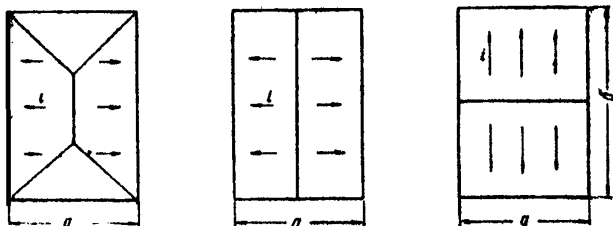
Рис. 2. Уклоны поверхности площадок для ручных спортивных игр i = 0,002 - 0,005
