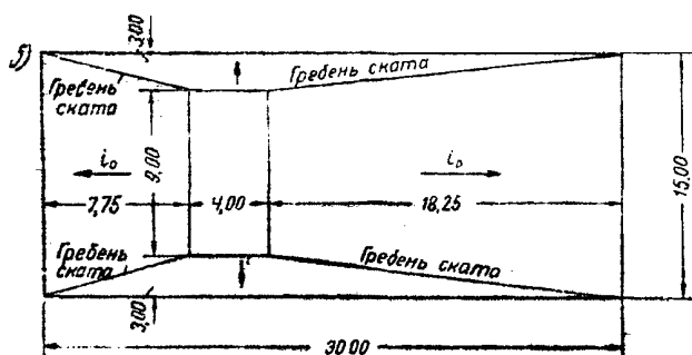
а—план; б—схема планировки поверхности площадки; i_0 = от 0,002 до 0,005
