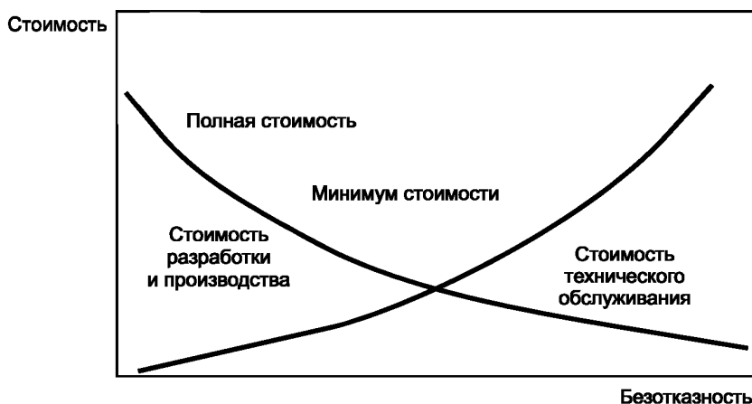
Рисунок 1 — Зависимость стоимости от безотказности
