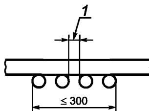
1 — зазор
