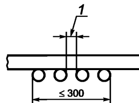
1 — зазор
