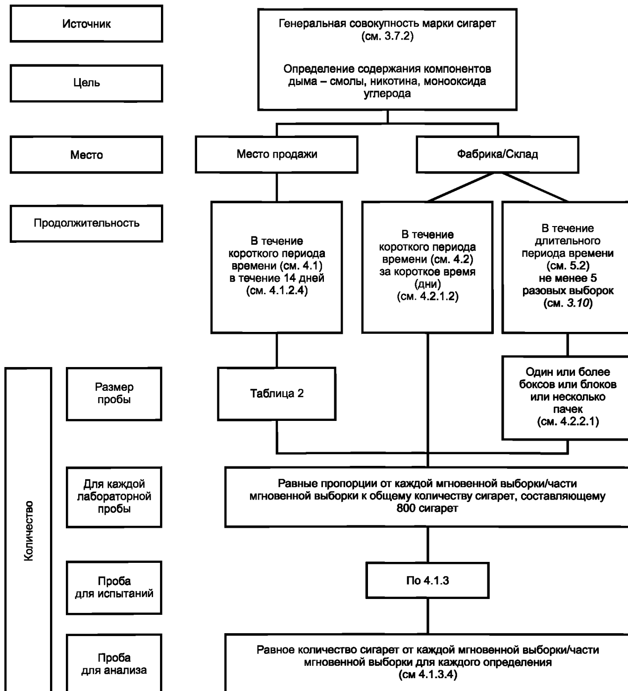
Рисунок А.1 — Схема отбора проб сигарет
