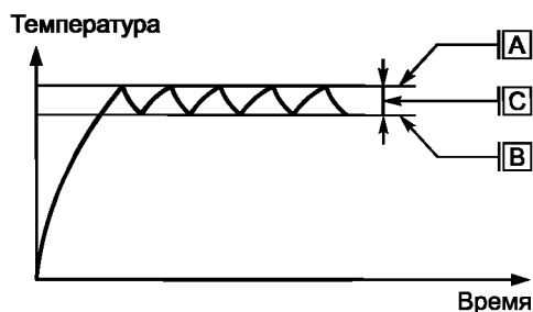
A — верхняя температура; B — нижняя температура; C — дифференциал
