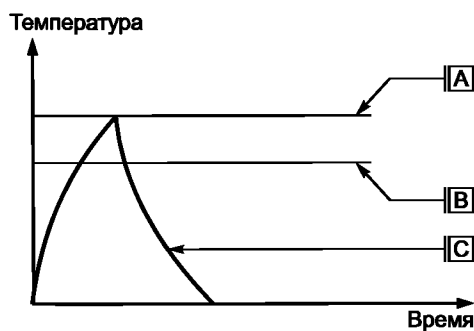
A — установленная температура; B — температура перезапуска; C — требуется ручной перезапуск
