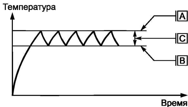
A — верхняя температура; B — нижняя температура; C — дифференциал (обычно значительно больше, чем у терморегулятора)
