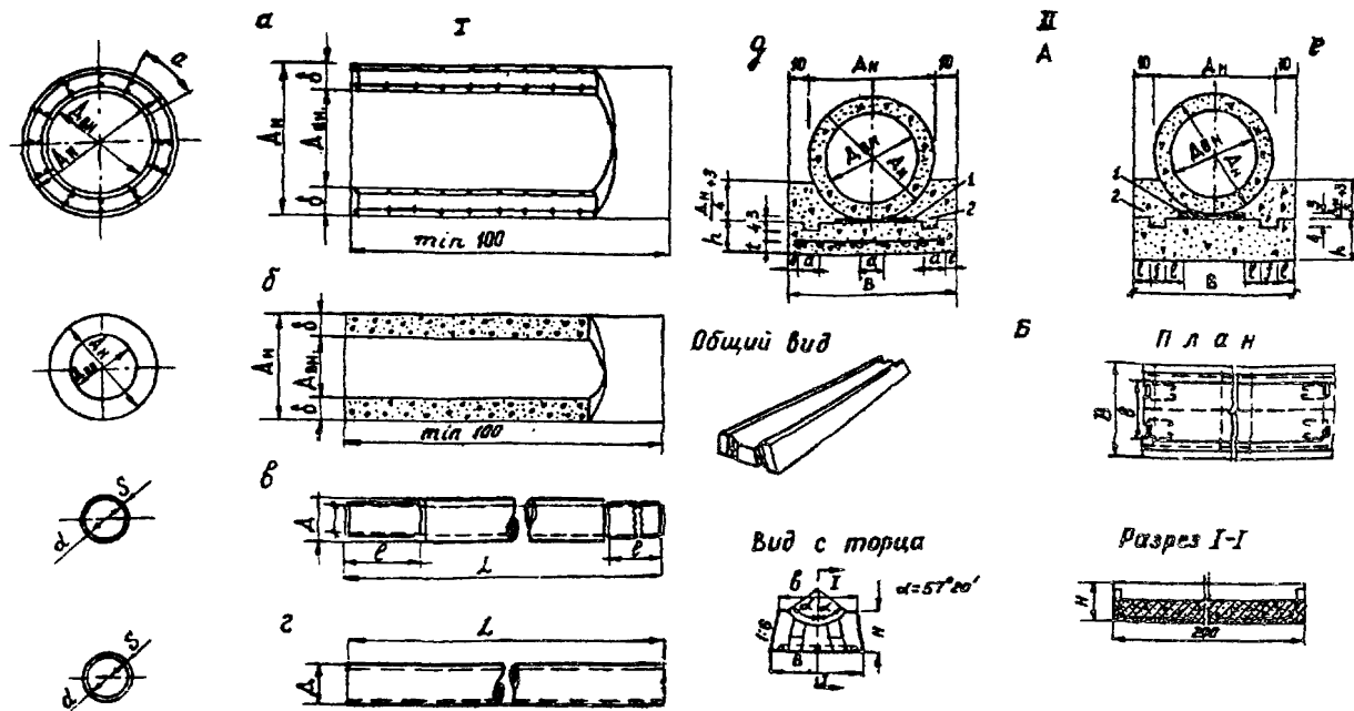
Рис. II. Трубы и основания под трубы: I- трубы для водосточков: а- железобетонные, б- высокопрочные бетонные, в- асбестоцементные для напорных трубопроводов, г- асбестоцементные для безнапорных трубопроводов; II- основания под высокопрочные бетонные и железобетонные трубы: А- монолитные: д- железобетонное, е- бетонное; Б- блоки сборного основания: 1- цементный раствор; 2- бетон
