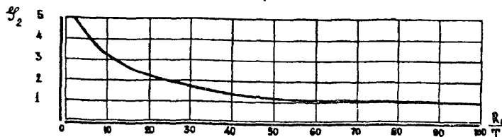
График функции F(\frac{r_0}{T}) для определения положения кривой депрессии в центре кольцевой дренажной сети
