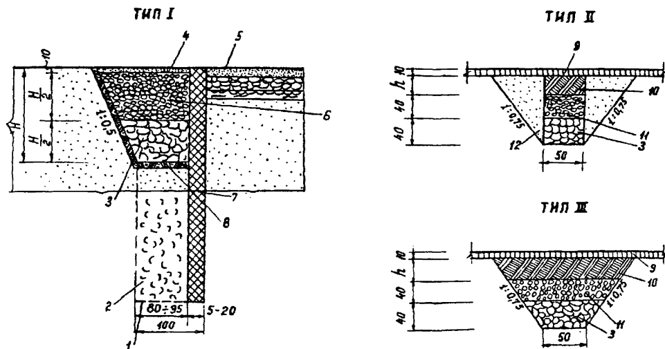
Рис.17. Конструкции дренажей и экранирующих устройств в вечномерзлых грунтах:
