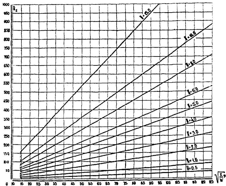
Рис. II. График для определения радиуса депрессии линейного дренажа при установившемся движении грунтовых вод R_2 м ( по формуле : R_2 = h \sqrt{\frac{K}{2W}} )
