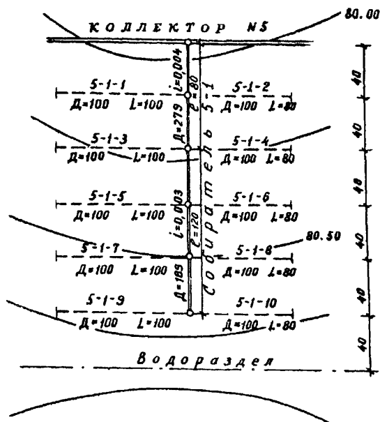
Рис.5. Схема собирателя 5-I (пример)
