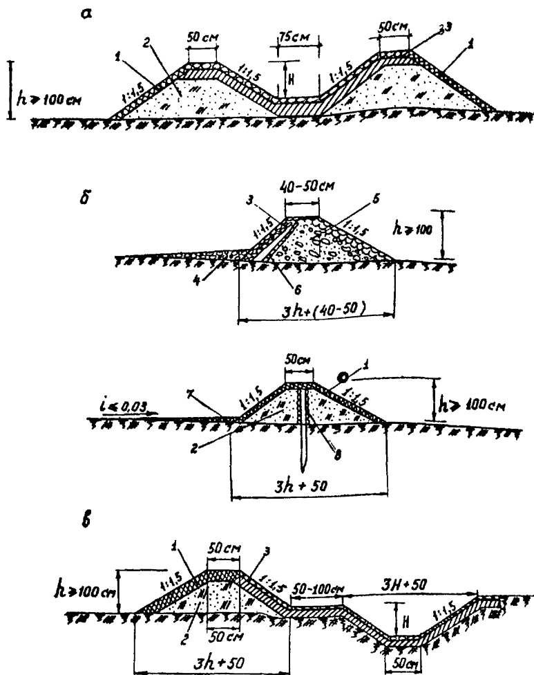
Рис.16. Конструкции элементов водоотводных сетей на вечноммерзлых грунтах:
