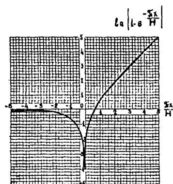
Рис.12. График для определения значения \ln|1 - e^{-\frac{x}{H}}| при вычислении ординат депрессионной кривой ( H_{\Sigma} ) в однолинейных дренажах несовершенного типа
