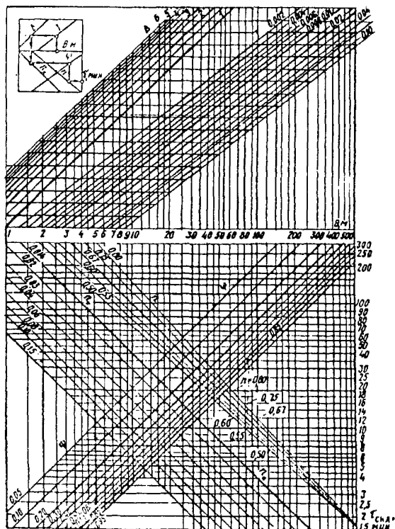
Рис.2. Номограмма для определения времени добрегания дождевых вод по склону \alpha (в мин)
