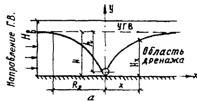
Рис.9. Расчетные схемы глубинного дренажа: А- систематический; Б- кольцевой (контурный); В- однолинейный; а- совершенный; б- несовершенный
