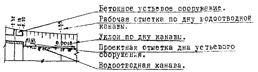
Рис.20. Продольный профиль по коллектору (пример оформления рабочих чертежей)
