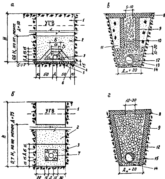
Рис.7. Поперечные сечения дрен и осушителей (размеры даны в сантиметрах):
