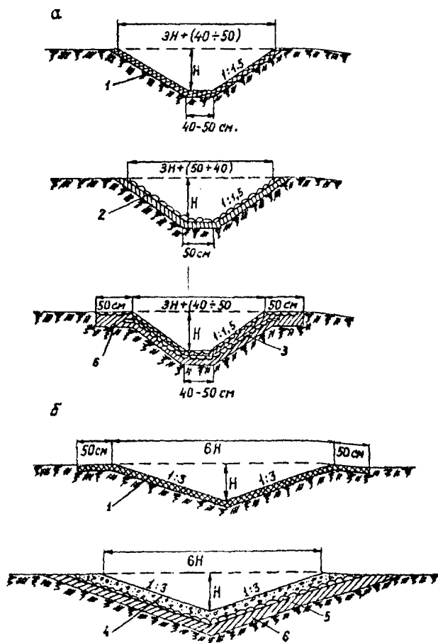
Рис.15. Конструкции элементов водоотводных сетей на вечномерзлых грунтах:
