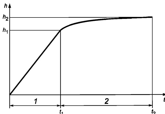
Рисунок А.3 — Ползучесть при индентировании
