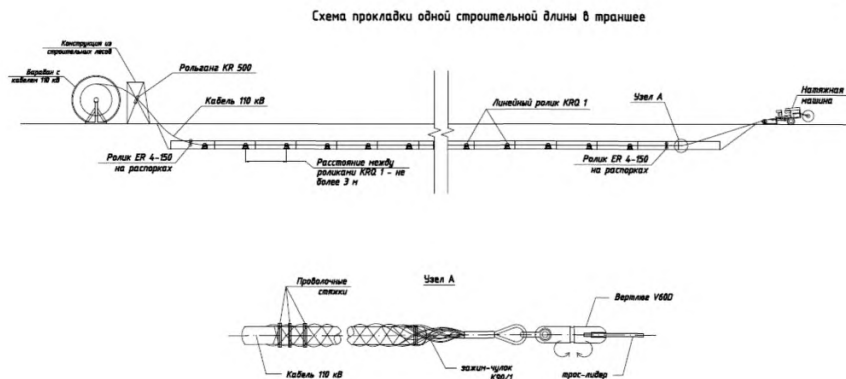
Рис.4 Протяжка кабеля
