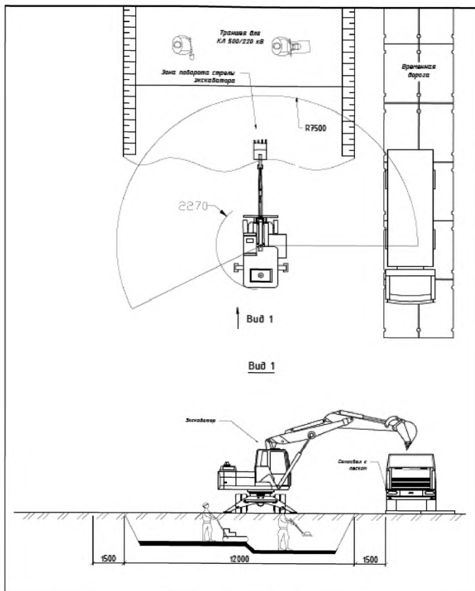
Рис. 1 Раскопка траншеи, устройство песчаной подушки с тронбровкой
