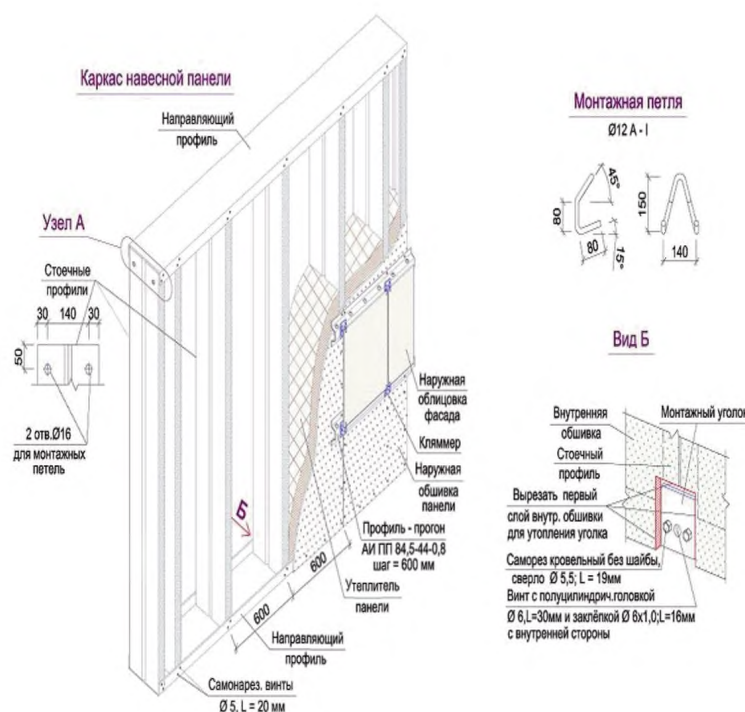
Рис2. Состав панели
