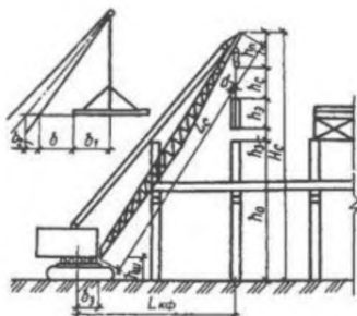
Рис.4. Схема параметров для выбора монтажного, стрелового самоходного крана
