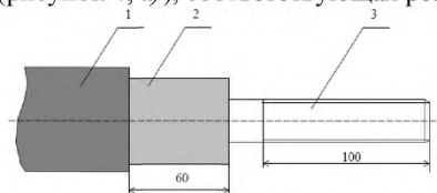
1 – наружная оболочка, 2 – изоляция, 3 – токопроводящая жила а) разделка кабеля с однопроволочной жилой при тяжении за жилу
