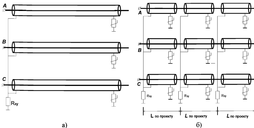
Рисунок 1 – Варианты одностороннего заземления экранов на КЛ
