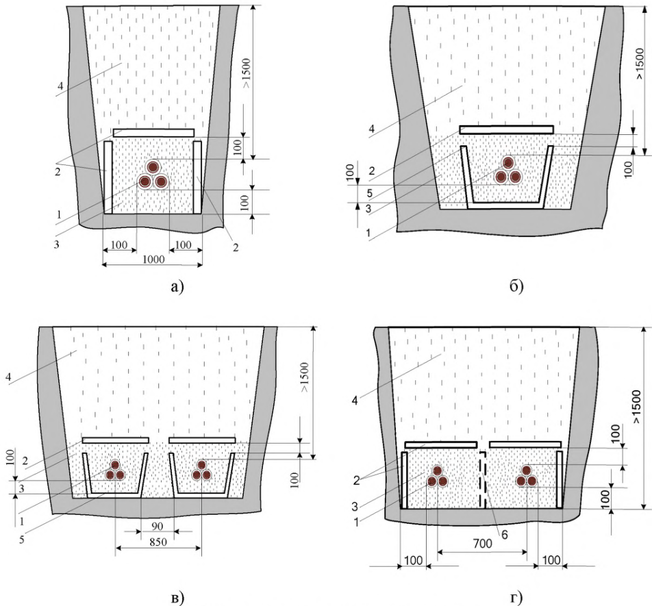
в) 1 – кабель, 2 – железобетонная защитная плита, 3 – песчано-гравийная смесь (толщина стабилизированного грунта принимается по проекту), 4 – засыпной грунт, 5 – железобетонный лоток, 6 – дополнительная железобетонная плита (согласно проекту) Рисунок И.1 – Примеры прокладки кабелей в траншеях
