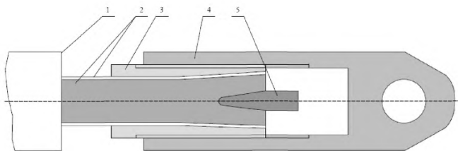
1 - кабель, 2 – жила кабеля, 3 – втулка, 4 – приспособление для тяжения, 5 – клин в) клиновый захват для тяжения кабеля с однопроволочной жилой Рисунок 4 - Протяжка кабеля с помощью концевой и клинового захвата
