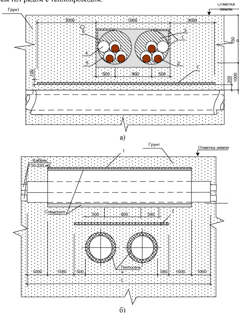
1 – железобетонные плиты В-4 (500х500х50), 2- кабель, 3 – бетонный раствор, 4 – резервная полиэтиленовая труба, 5 - полиэтиленовые трубы из ПНД диаметром 225 мм, 6 – стальная труба диаметром 710 мм, 7- дополнительная теплоизоляция из пенополистирольных плит (толщиной по проекту), покрытых гидроизолом Рисунок И.3 – Пример прокладки кабелей 110 (220) кВ над теплосетью в поперечном
