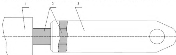
1 – кабель, 2 – жила кабеля, 3 – приспособление для тяжения б) концевой захват для тяжения кабеля с многопроволочной жилой
