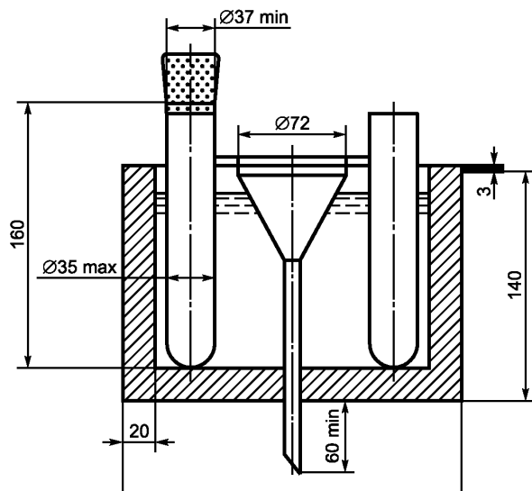
Рисунок 2 — Охлаждающая баня
