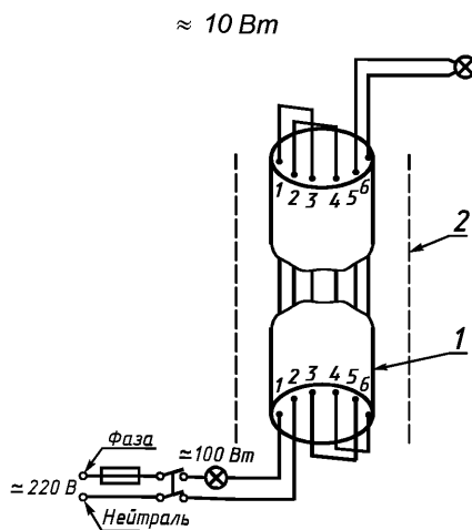
Рисунок 6 — Электрическая схема для испытания на нераспространение горения
