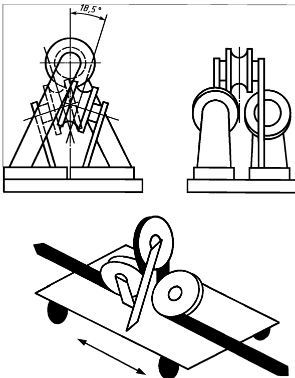
Рисунок 4 — Модифицированная каретка
