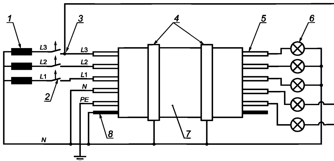
1 — трансформатор; 2 — плавкий предохранитель (2 А); 3 — подсоединение к фазе (или L1, или L2); 4 — поддерживающие кольца; 5 — испытываемая жила или группа жил; 6 — нагрузочный индикаторный прибор (например, лампа); 7 — образец; 8 — металлический экран (если имеется); L1, L2, L3 — фазные жилы (L2, L3, если имеются); N — нейтральная жила (если имеется); PE — защитная жила (если имеется)
