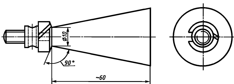
Рисунок 1 — Коническая оправка
