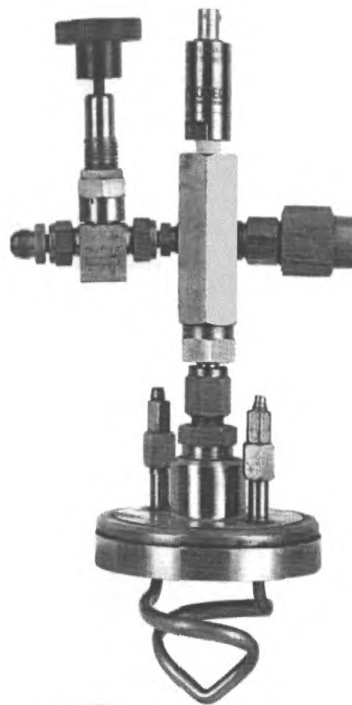
Рисунок 3 — Крышка с охлаждающим змеевиком
