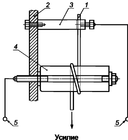
1 — образец; 2 — изоляционный материал; 3 — верхний зажим; 4 — цилиндр; 5 — испытательное напряжение
