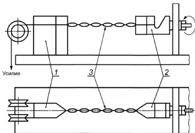
1 — неподвижная распорка; 2 — вращающийся крюк-распорка; 3 — образец Рисунок 2 — Устройство для скручивания образца для испытания пробивным напряжением
